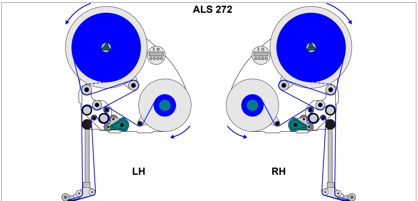
[36] Esquema de enhebrado para ALS 272 con borde de dispensadora L
