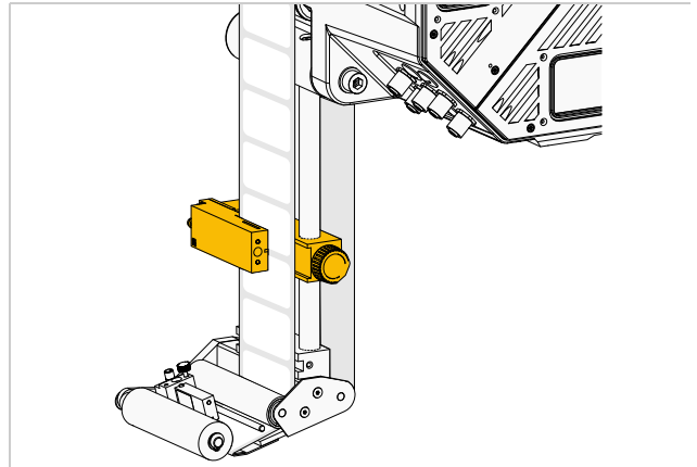
[20] Sensor capacitativo.
