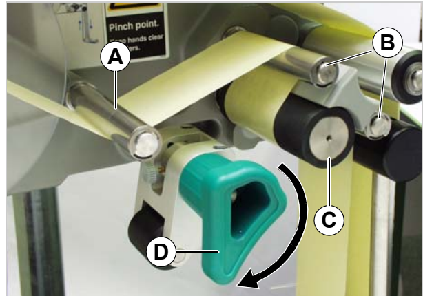
[41] Abrir el rodillo de presión.
