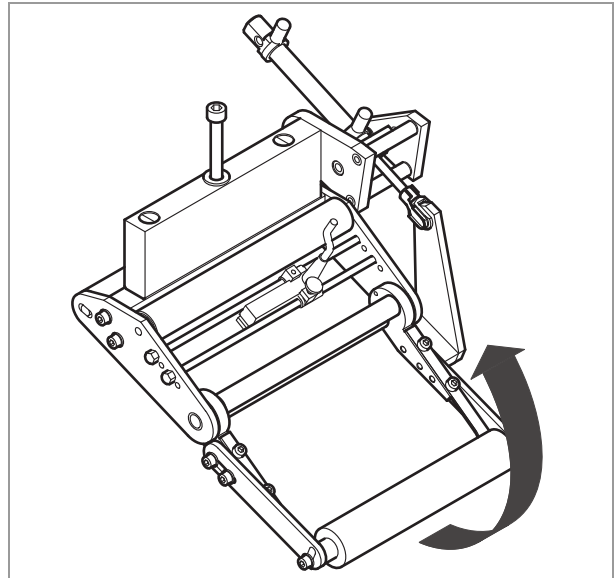
[14] Borde de salida neumático
