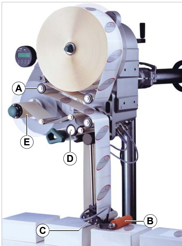
[4] Etiquetadora ALS 20x preparado para el servicio.
