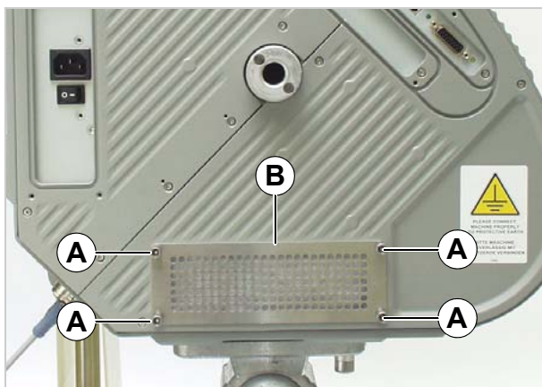
[60] Filtro de polvo en el ALS 256/ALS 272.
