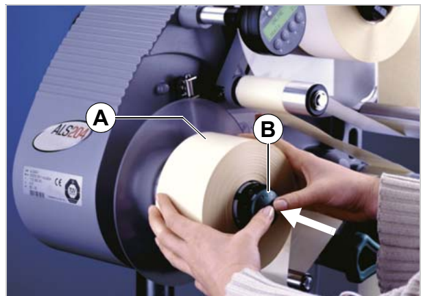
[33] A Papel de soporte enrollado B Botón de desbloqueo
