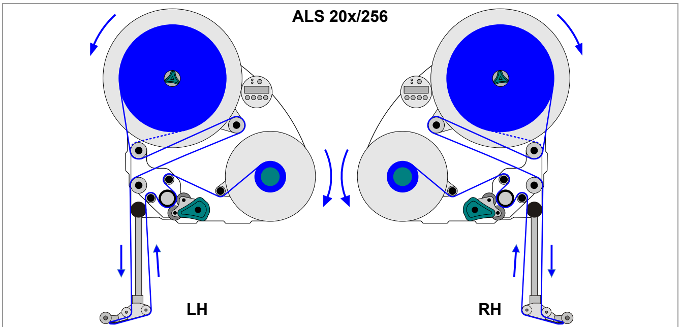
[35] Esquema de enhebrado para ALS 20x/256 con borde de dispensadora L
