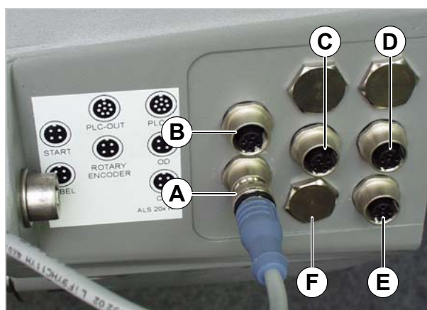
[32] Conexiones de los sensores:
