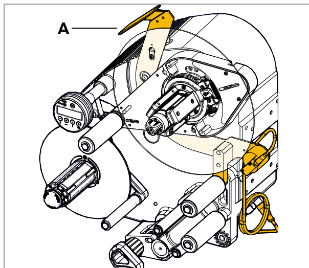
[17] Barrera óptica DR (A)
