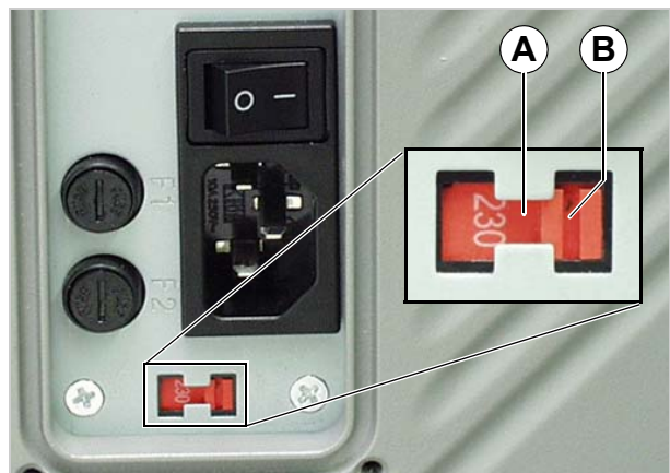
[30] Selector de tensión (ajuste en la ilustración: 230 V)
