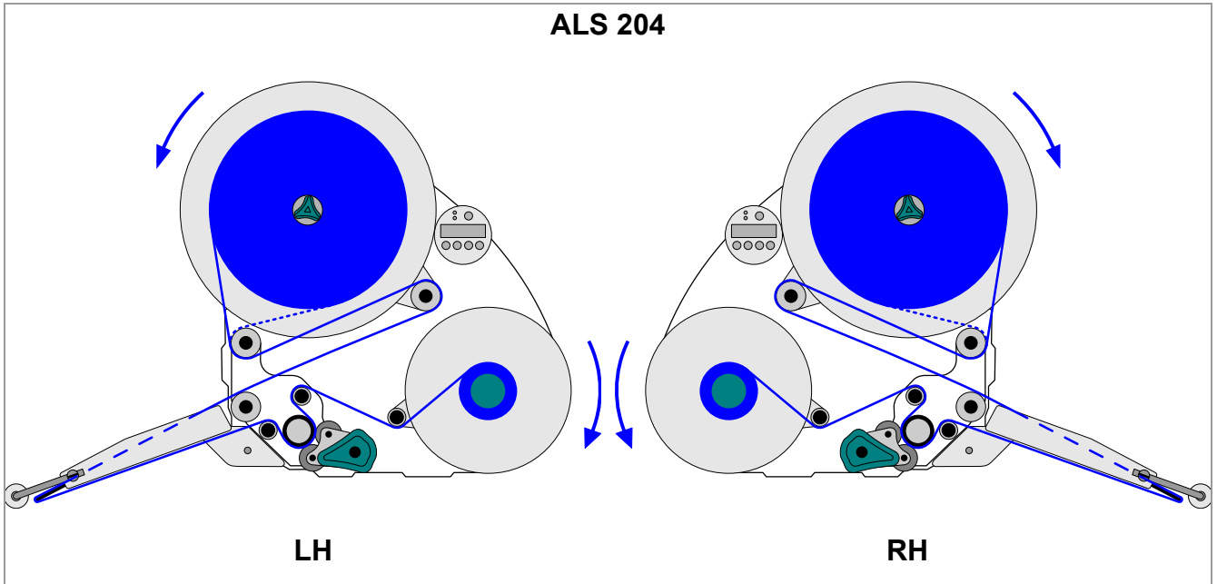
[37] Esquema de enhebrado para ALS 20x/256 con borde de dispensadora V
