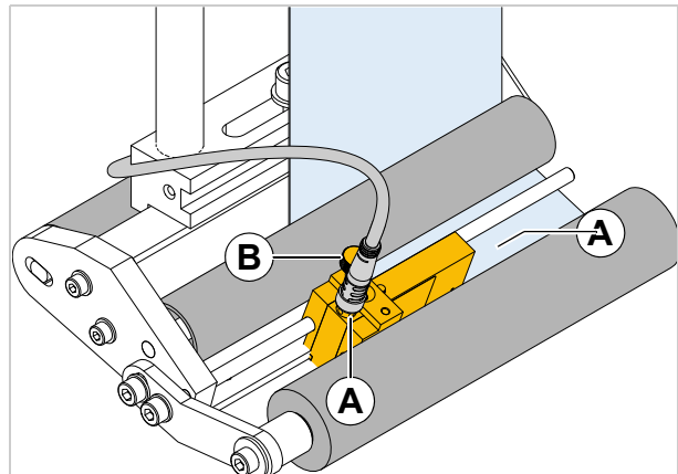
[47]] Fotocélula de etiquetas en borde dispensador L fijo.
