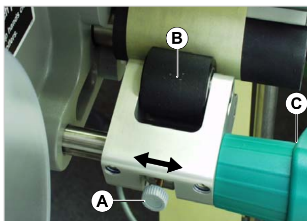
[46] Ajustar la posición del rodillo de presión (B).
