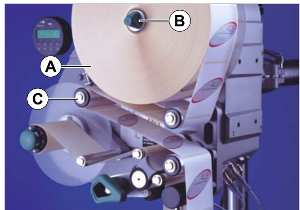
[34] Introducir rollos de material - Parte 1
