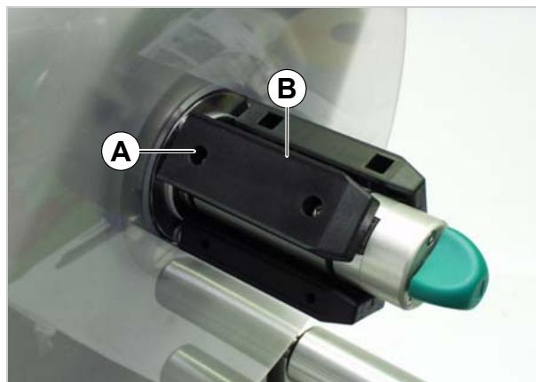
[44] Posición del adaptador de núcleos para un diámetro de núcleo de 76,2 mm.
