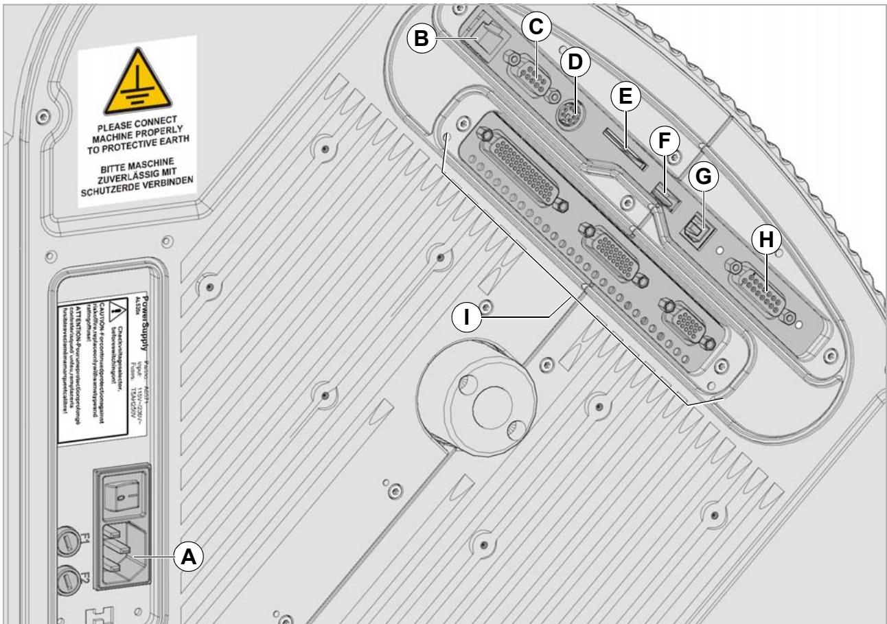
[7] Conexiones en la parte posterior de la máquina (ALS 20x)
