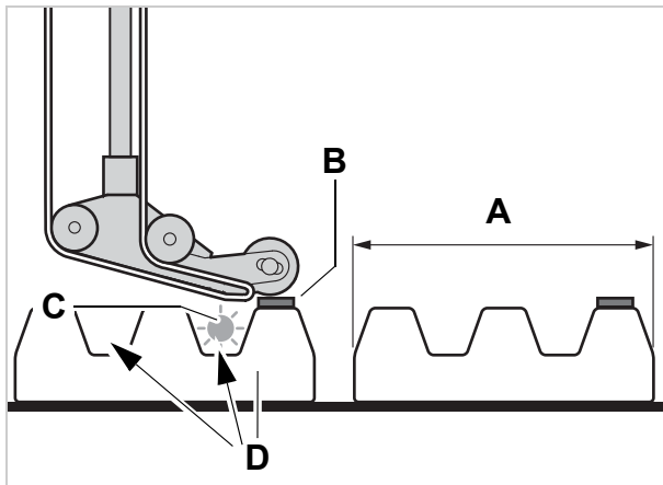
[53] A Longitud Producto B Etiqueta C Sensor de producto D Producto con entalladuras (flechas)
