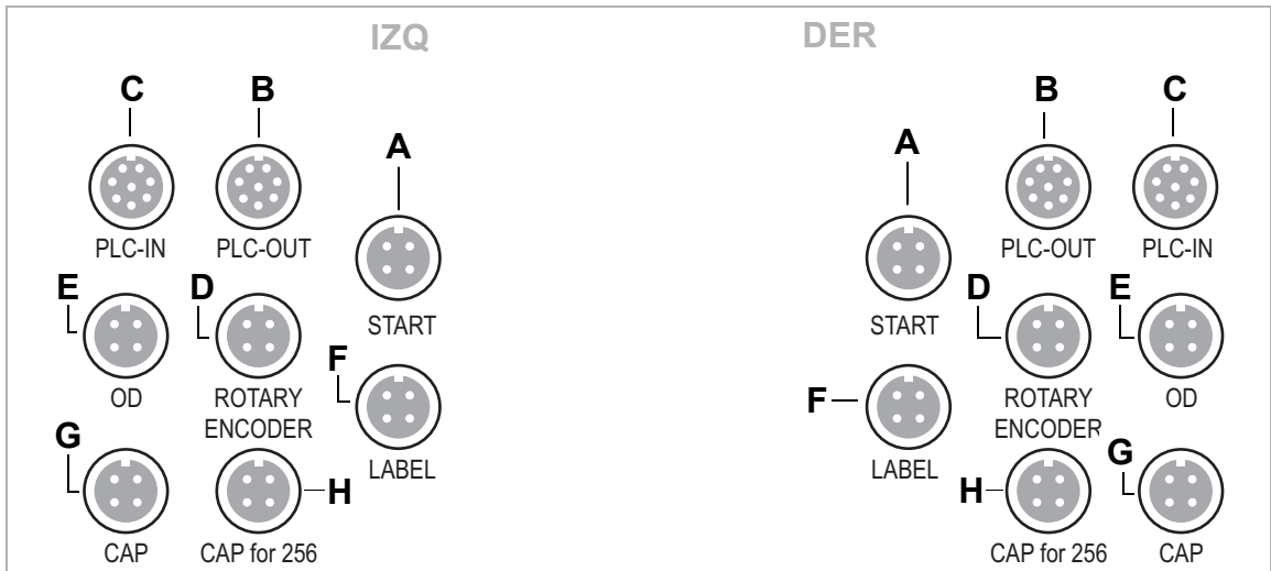
[8] Conexiones de los sensores del ALS 20x (DER)
