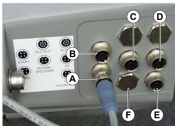
[31] Conectores para sensores:
