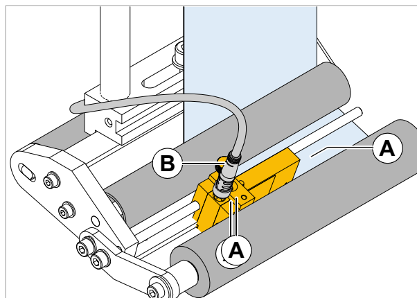
[46] Célula fotoeléctrica de etiquetas na borda fixa de dispensa L.
