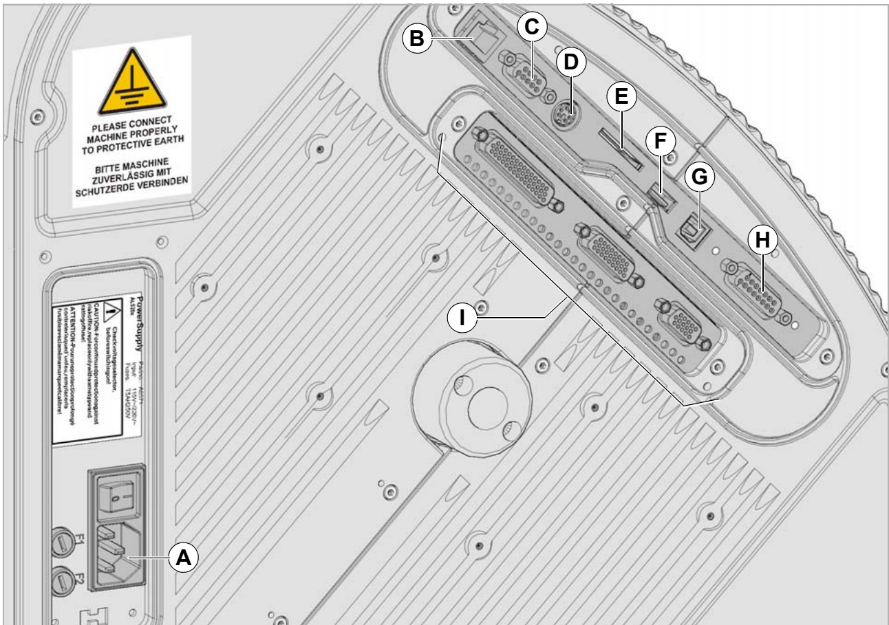
[6] Conectores no painel traseiro do aparelho (ALS 20x)
