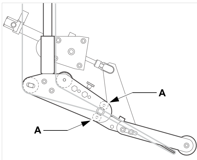
[39] Decurso da fita de etiquetas na borda dispensadora pneumática (opcional).
