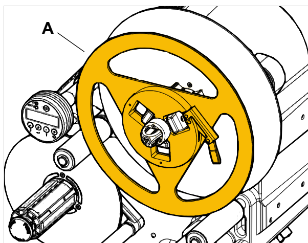
[18] Disco de guia adicional do material (A)
