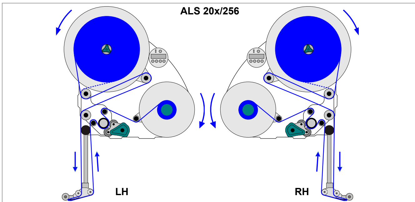
[34] Esquema de introdução para a ALS 20x/256 com borda dispensadora tipo L.
