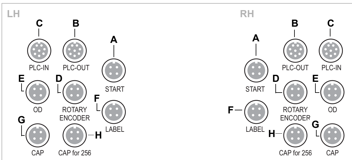
[8] Disposição (esquemática) dos conectores para sensores em máquinas de versão esquerda LH (Fig. à esquerda) e máquinas de versão direita RH (Fig. à direita):
