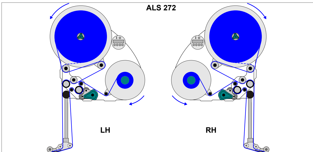
[35] Esquema de introdução para a ALS 272 com borda dispensadora tipo L.
