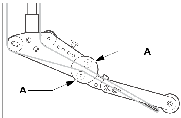
[38] Decurso da fita de etiquetas na borda dispensadora amortecedor (opcional).
