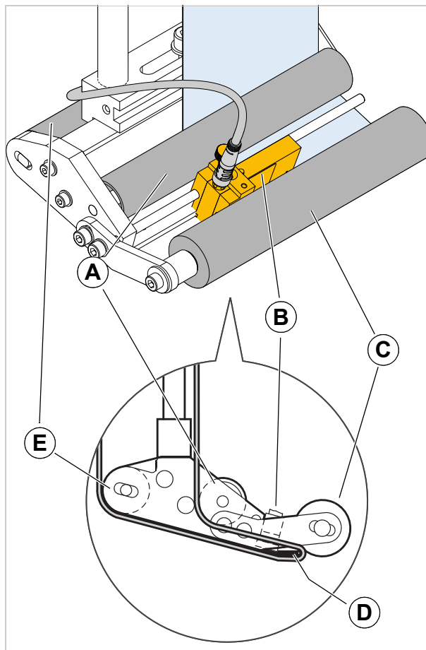
[37] Decurso da fita de etiquetas na região da borda dispensadora.
