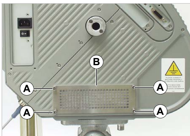
[59] Filtro do pó no ALS 256/ALS 272.
