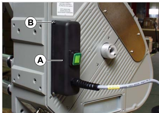
[28] ALS 20x com protecção contra água respingada: Primeiramente, remover a concha de cobertura (A).
