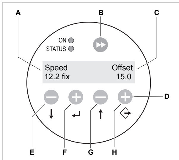
[24] Painel de operação no modo de operação Ajustes Online.
