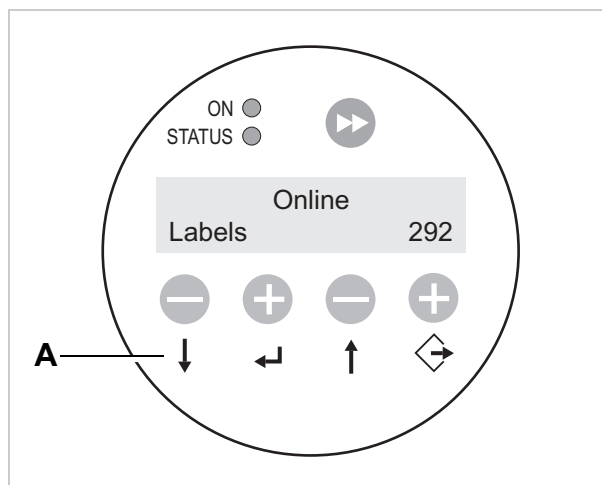
[23] Painel de operação durante a operação de dispensa (292 etiquetas dispensadas)
