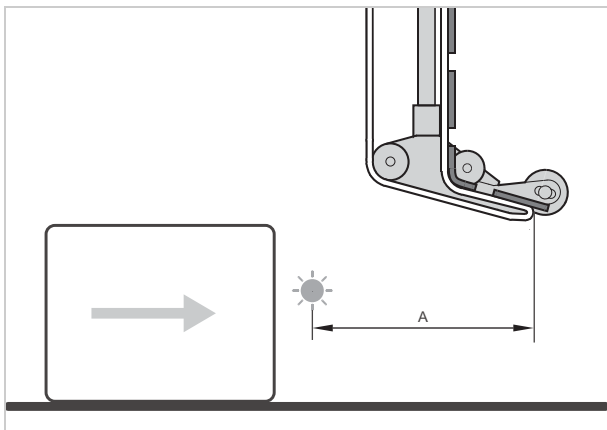
[53] Distância entre o detector fotoelétrico de produto (à esquerda) e a borda dispensadora (à direita).
