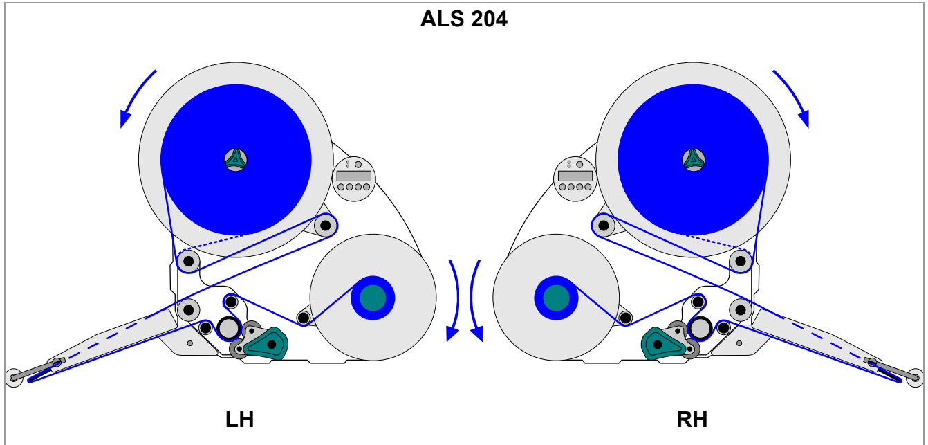
[36] Esquema de introdução para a ALS 204 com borda dispensadora tipo V.
