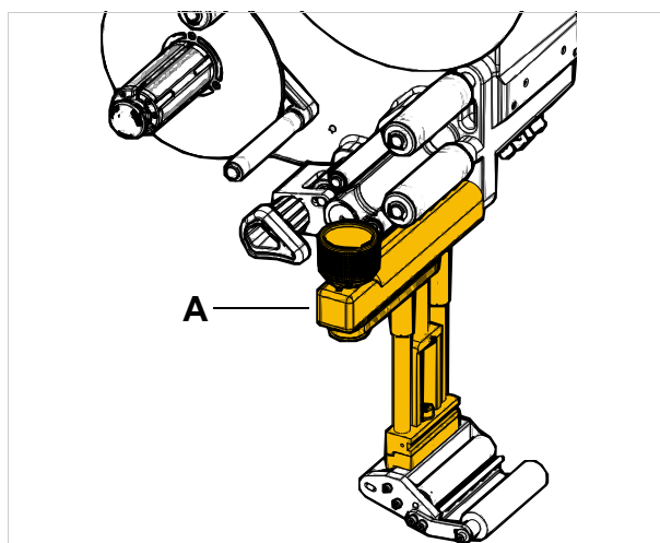
[15] Suporte da borda dispensadora ajustável (A)
