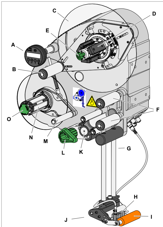
[4] Etiquetador ALS 204 versão direita
