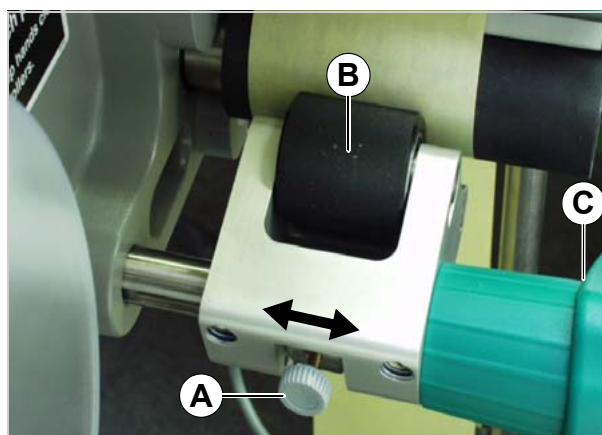
[45] Ajustar a posição do rolo de pressão (B).
