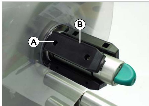
[43] Posição do adaptador de tubo para diâmetro de tubo de 76,2 mm.
