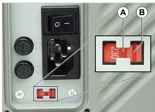
[29] Selector de tensão (ajuste na Fig: 230 V)
