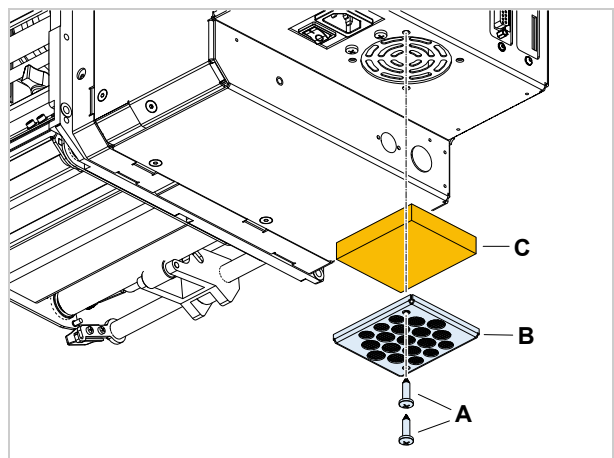
[73] Filtergehäuse abgenommen.
