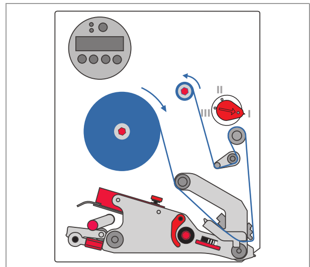
[42] Fädelschema für Folie.
