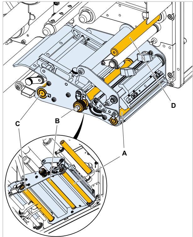
[63] Positionen der Gummwalzen am DPM:
