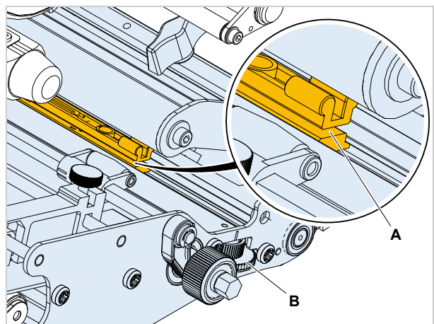
[68] Lichtschrankengabel (A).
