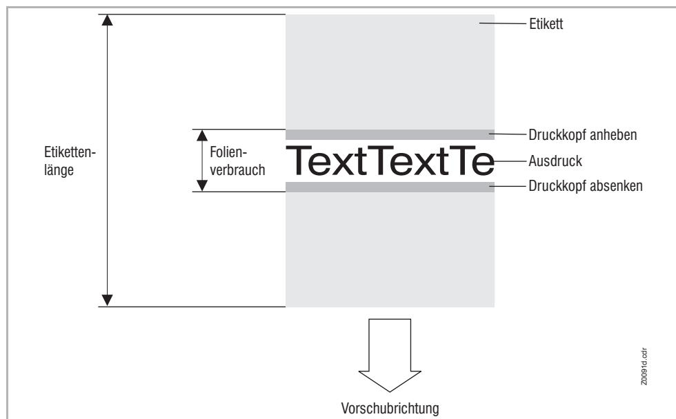
[17] Folienverbrauch für Etiketten mit kleinem Druckbereich bei eingeschalteter Folienspar-Automatik. Der Folienverbrauch ist geringfügig höher, als die Länge des bedruckten Bereichs.
