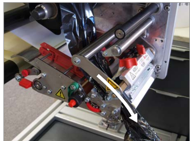
[43] Folie seitlich am Druckkopf einfädeln.
