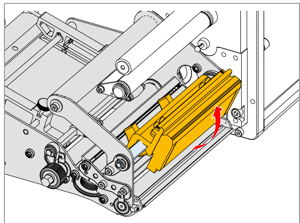
[56] Druckkopf hochschwenken.
