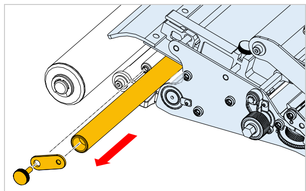
[66] Umlenkrolle herausziehen.
