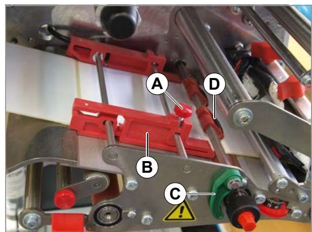
[34] Materialführung einstellen.
