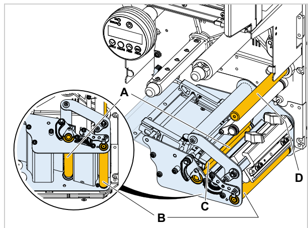
[64] Positionen der Gummwalzen am PEM:
