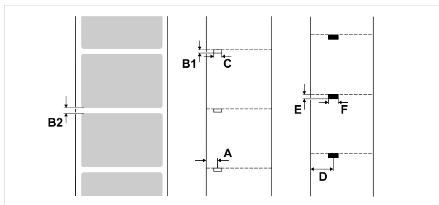
Image 9: Dimensions et positions des estampages et des repères type réflex ( A : Position d'estampage, B : Longueur d'estampage, C : Largeur d'estampage, D : Position des repères type réflex, E : Longueur des repères type réflex, F : Largeur des repères type réflex).
