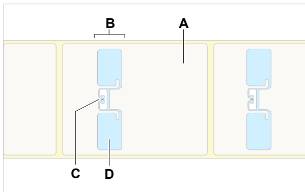
Image 5: Schéma d'une étiquette RFID (A : étiquette, B : transpondeur, C : puce, D : antenne)
