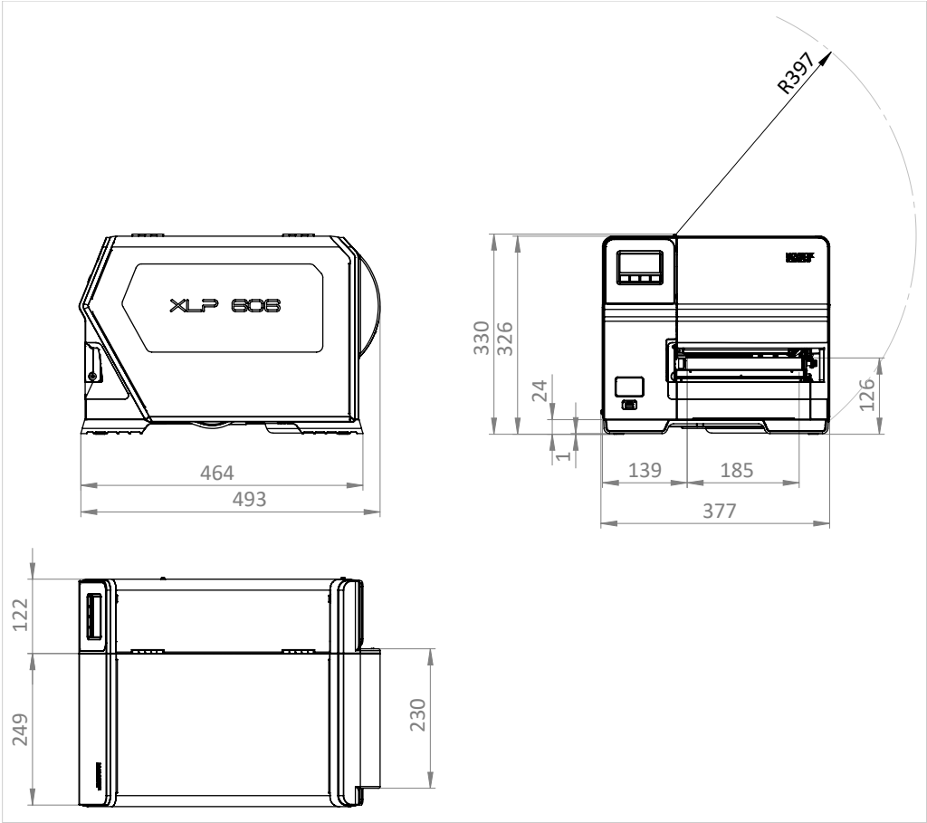
Image 7: Dimensions du XLP 605/606.
