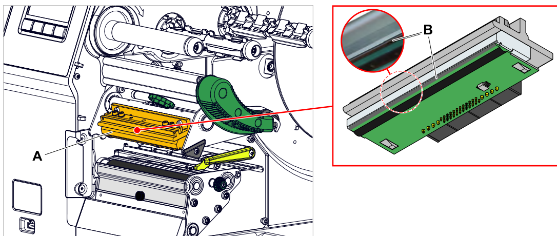
Image 68: A : tête d'impression, B : barre thermique sur la tête d'impression
