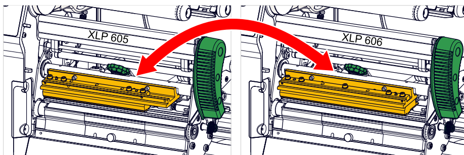
Image 69: Les têtes d'impression XLP 605 et XLP 606 peuvent être interchangeables. La tête d'impression montée est détectée automatiquement et les réglages pertinents sont adaptés.
