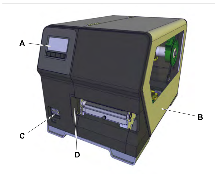
Image 15: Éléments de commande à l'extérieur du XLP 604 Peripheral.
