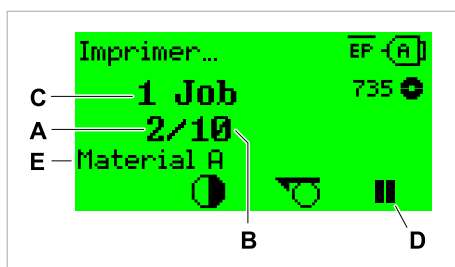
Image 55: Affichage pendant l'impression (A : étiquettes déjà imprimées de la tâche d'impression actuelle, B : étiquettes à imprimer de la tâche d'impression, C : nombre de tâches d'impression dans la file d'attente, D : touche Pause, arrête l'imprimante, E: (Facultatif) Nommer le matériel d'impression, voir la commande Easy Plug #IM).
