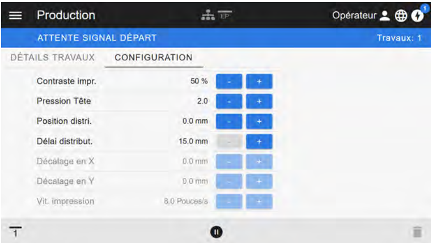
Image 27: Vue « Configuration » d'une tâche d'impression dans le panneau Web. Des configurations inaccessibles avec le rôle activé (dans notre exemple : « Opérateur ») sont affichées en grisé. Les autres configurations peuvent être modifiées en cliquant sur « + » ou « - ».
