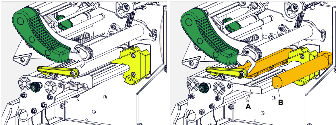
Image 4: À gauche : XLP 604 sans RFID ; à droite : XLP 604 avec RFID (A : antenne ; B : brosse antistatique).
