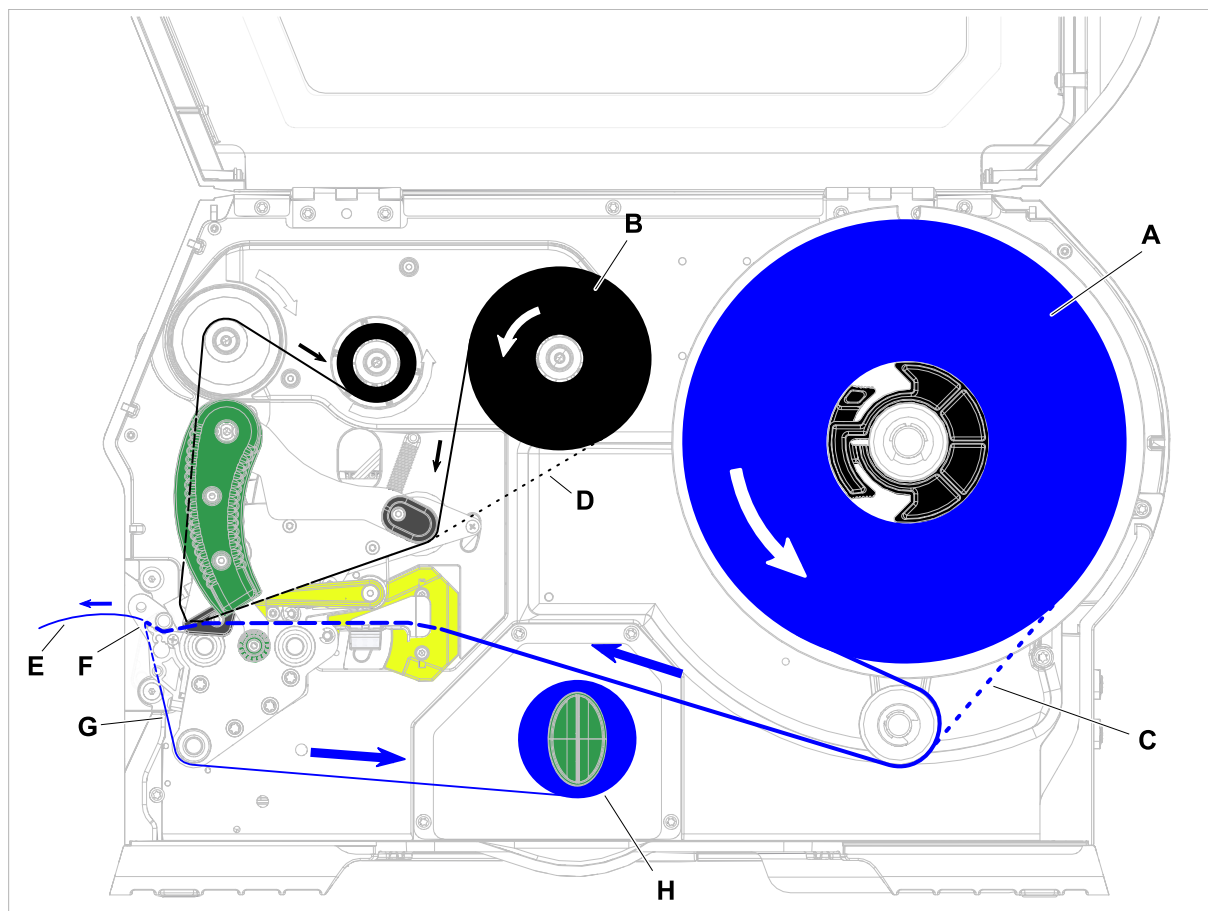
Image 44: Croquis d'insertion pour XLP 60x Dispenser. A: Rouleau d'étiquettes, B: Rouleau de ruban transfert, C: chemin pour matériel d'étiquetage embobiné vers l'intérieur, D: chemin pour ruban transfert embobiné avec côté encre vers l'extérieur, E: Étiquette donnée, F: Plaque de pose, G: Dorsal étiquettes, H: Réenrouleur interne
