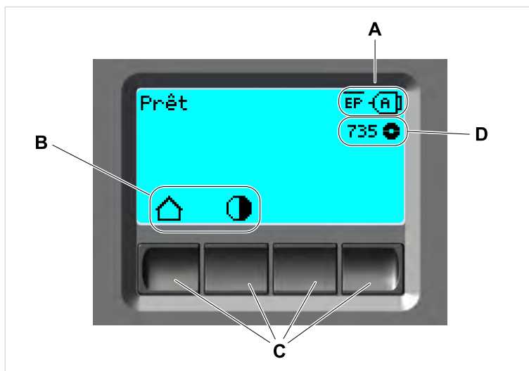
Image 20: Éléments sur le panneau de commande du XLP 60x: A Icônes fournissant des informations sur l'affectation des interfaces, B Icônes indiquant l'affectation des touches, C Touches de commande, D Affichage de la réserve de ruban transfert.
