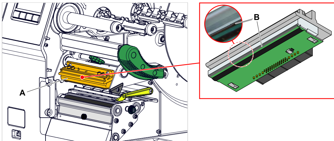
Image 64: A : tête d'impression, B : barre thermique sur la tête d'impression
