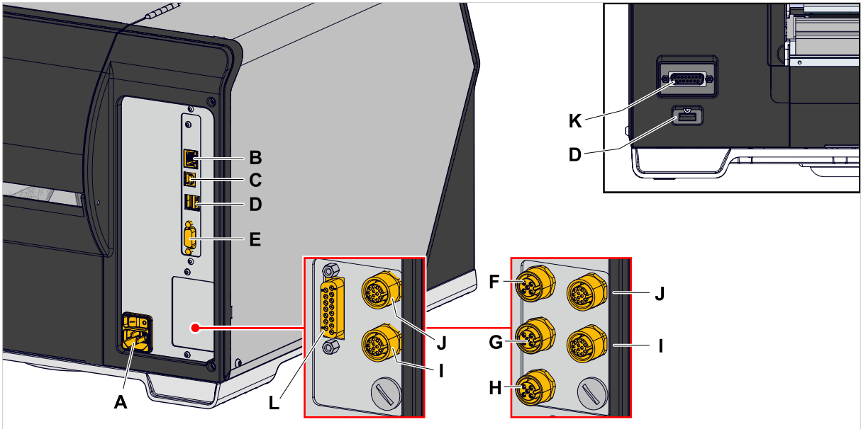
Image 36: Prises d'un XLP 60x Peripheral, en option avec des platines d'interface « BasicIO » (F-H) et « 8IO » (I, J) ou avec des platines d'interface « Basic-USI » (L) et « 8IO » (I, J).
