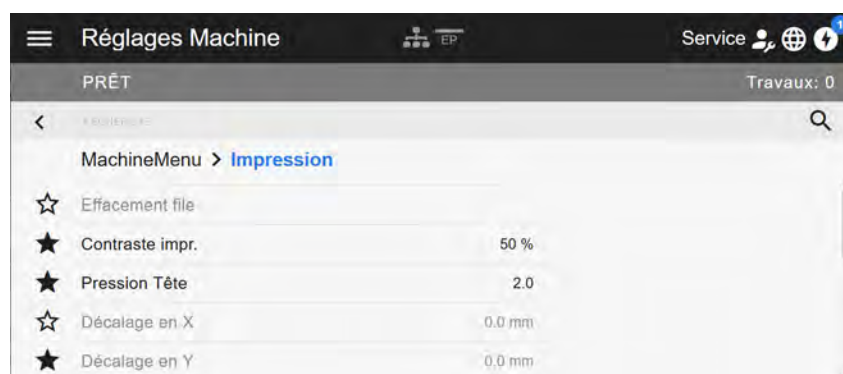
Image 35: Vue Configuration de la machine dans le panneau Web. Les étoiles à gauche à côté des paramètres marquent les favoris. Étoile remplie = paramètre sélectionné pour le menu Favoris.
