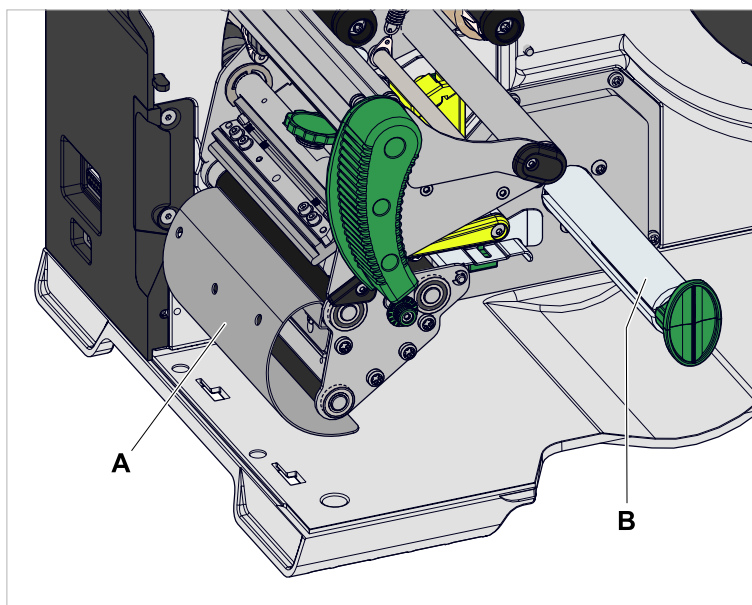
Image 17: Éléments de commande supplémentaires du XLP 60x avec enrouleur interne.
