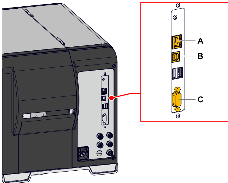
Image 37: Interfaces de données sur le XLP 60x (A Ethernet, B USB, C RS 232).
