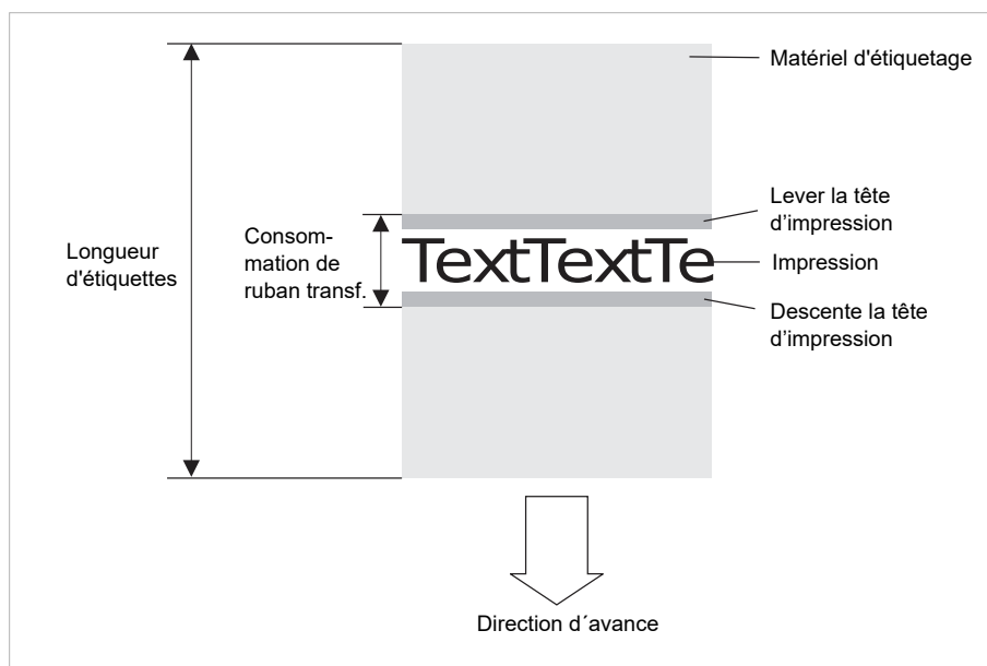
Image 14: Consommation de ruban transfert pour étiquettes avec petit domaine d'impression alors que l'automatisme d'économie de ruban transfert est activé. La consommation de ruban transfert est légèrement plus élevée que la longueur du domaine imprimé.
