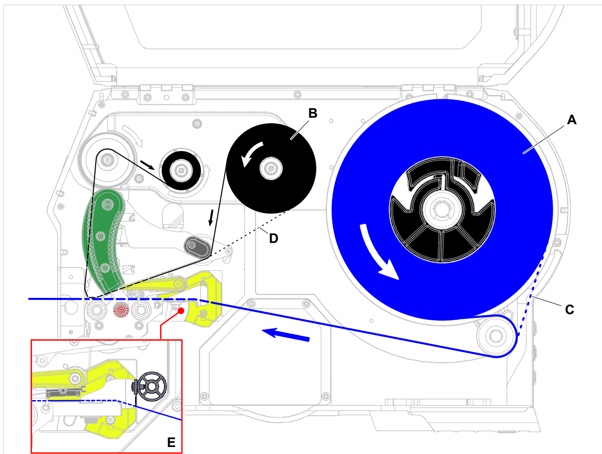
Image 43: Croquis d'insertion pour XLP 60x. A: Rouleau d'étiquettes, B: Rouleau de ruban transfert, C: chemin pour matériel d'étiquetage embobiné vers l'intérieur, D: chemin pour ruban transfert embobiné avec côté encre vers l'extérieur
