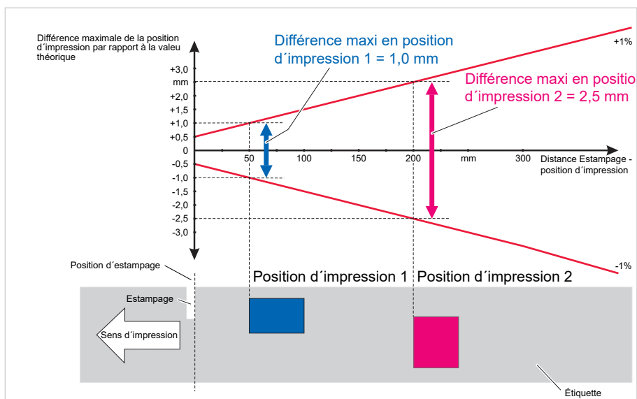
Image 10: La précision d'impression dépend de la position d'impression sur l'étiquette.
