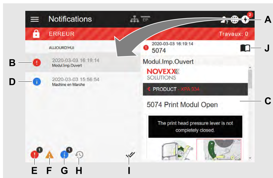
Image 24: La vue Notifications s'affiche après avoir cliqué sur le symbole de notifications (A). La partie gauche montre l'historique de notification, la partie droite montre une explication pour l'inscription sélectionnée dans l'historique.
