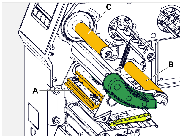
Image 66: Renvois du ruban transfert sur le XLP 60x (A: nez sur la tête d'impression, B: axes de renvoi, C: rouleau métallique ou rouleau en caoutchouc).
