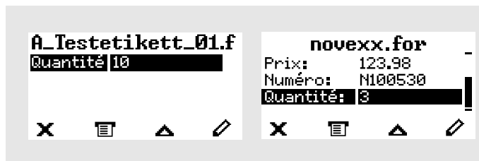
Image 53: Sélection de fichier en mode autonome (à gauche : champ standard pour interrogation de la quantité d'impression ; à droite : interrogation de données supplémentaires)
