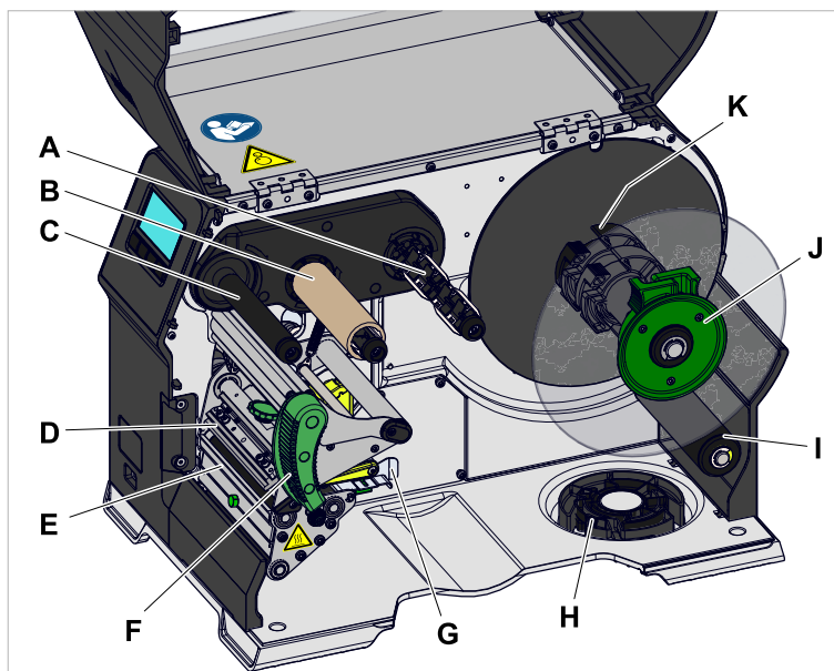
Image 16: Eléments de commande à l'intérieur du XLP 604.
