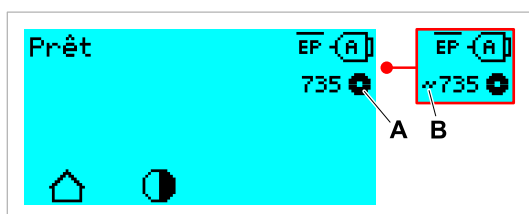
Image 49: Affichage de la longueur restante de ruban transfert (A, ici : 735 m).
