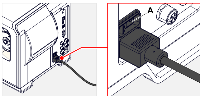
Image 38: Interrupteur d'alimentation (A) sur le XLP 60x.
