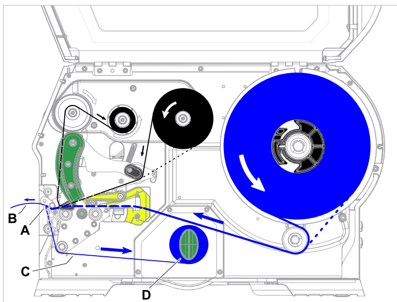
Image 13: Passage du matériel et du ruban transfert dans le XLP 60x avec enrouleur interne et plaque de distribution.
