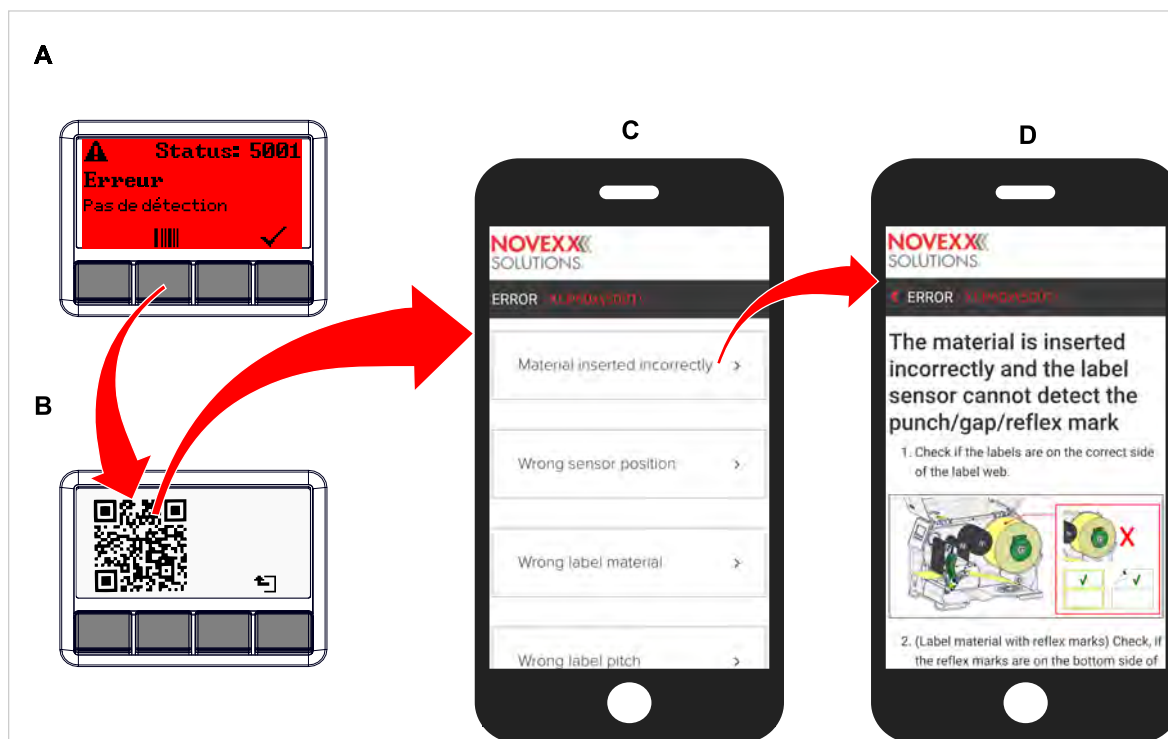
Image 63: Si le message d'erreur possède un symbole Code-barres (A), il est possible, par le biais d'un code QR (B) de faire afficher une notice pour l'élimination d'erreurs (C) sur le smartphone.
