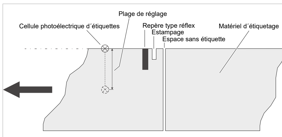
Image 11: Plage de réglage de la cellule photoélectrique d'étiquettes.
