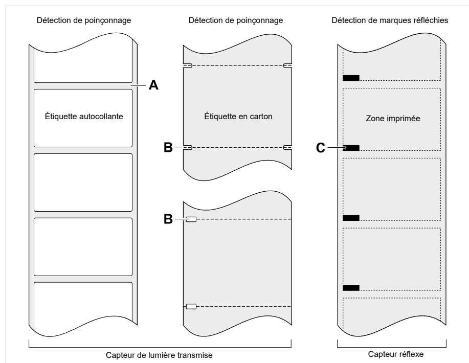
Image 70: Différents types et positions des repères de début d'étiquettes.
