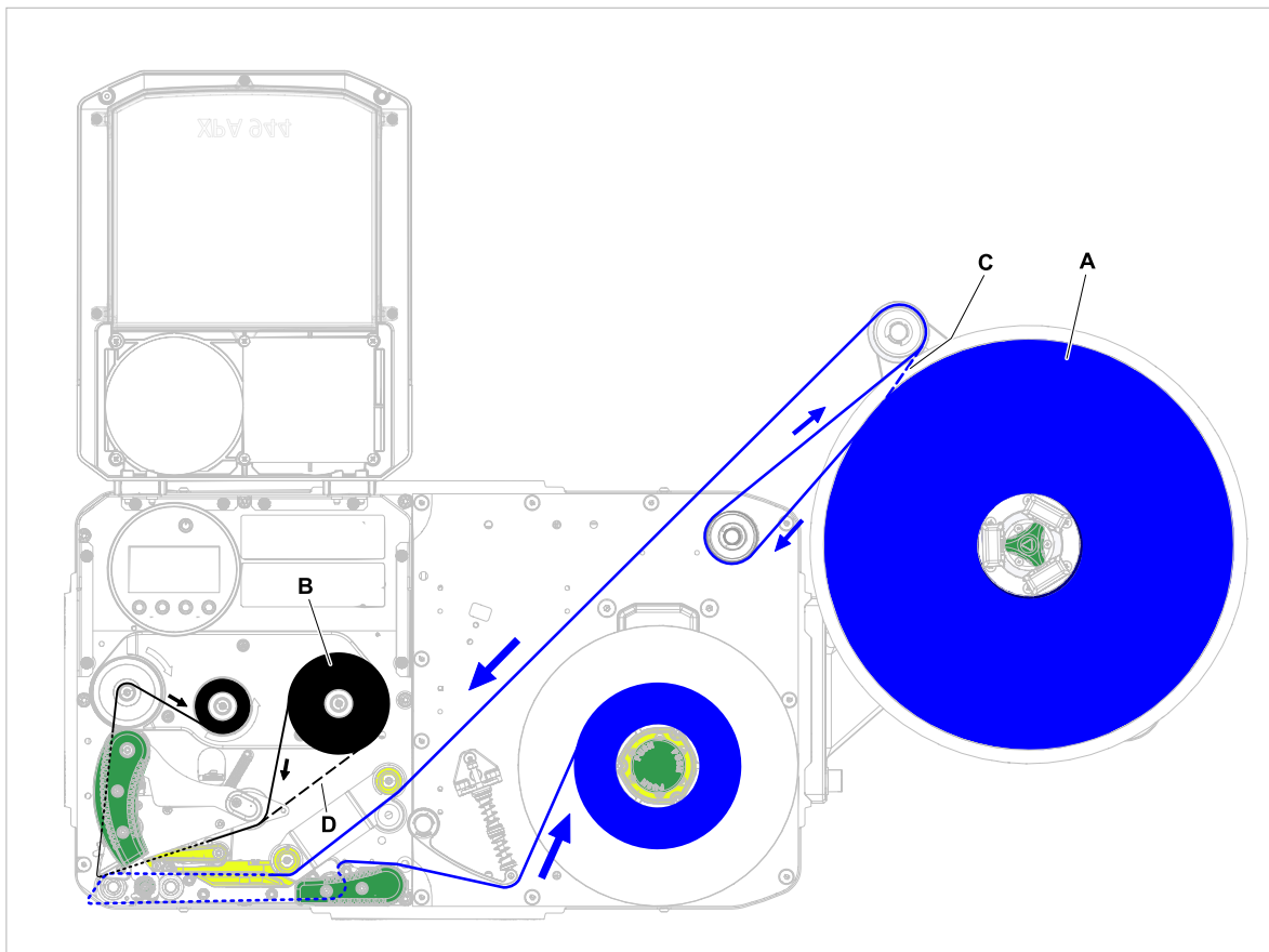
Figura 42: Esquema de enhebrado para el material de etiquetas (A) y lámina de termotransferencia (B) en el XPA 944 LH con desenrollador montado en el lado derecho . Con esta configuración es necesario un rodillo de inversión opcional para el material de etiquetas enrollado hacia el exterior. C = Camino del material de etiquetas enrollado hacia el interior; D = Camino de la lámina enrollada con el lado del color hacia el exterior.
