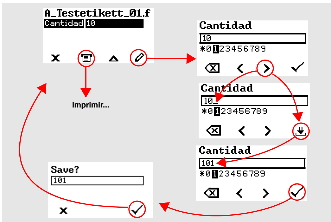
Figura 57: Modificar la cantidad de etiquetas en el modo standalone.
