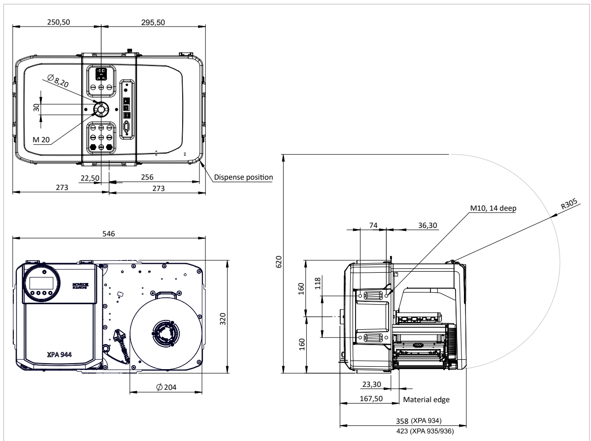
Figura 10: Dimensiones del XPA 944 LH.
