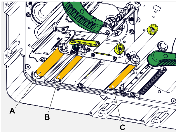
Figura 71: A Rodillo de impresión, B Rodillo de avance, C Rodillo de tracción
