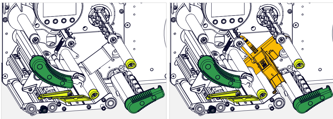
Figura 7: Izquierda: XPA 94x estándar; Derecha: XPA 94x con sensor de etiquetas transparentes.
