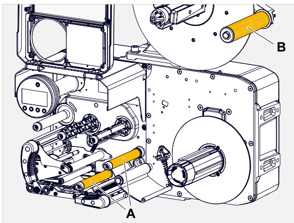
Figura 69: Ejes y rodillos de inversión en el XPA 944.
