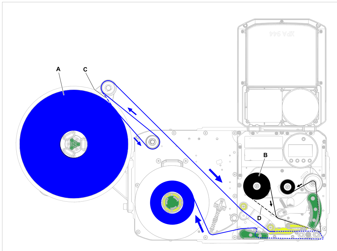
Figura 45: Esquema de enhebrado para el material de etiquetas (A) y lámina de termotransferencia (B) en el XPA 944 RH con desenrollador montado en el lado izquierdo . Con esta configuración es necesario un rodillo de inversión opcional para el material de etiquetas enrollado hacia el exterior. C = Camino del material de etiquetas enrollado hacia el interior; D = Camino de la lámina enrollada con el lado del color hacia el exterior.
