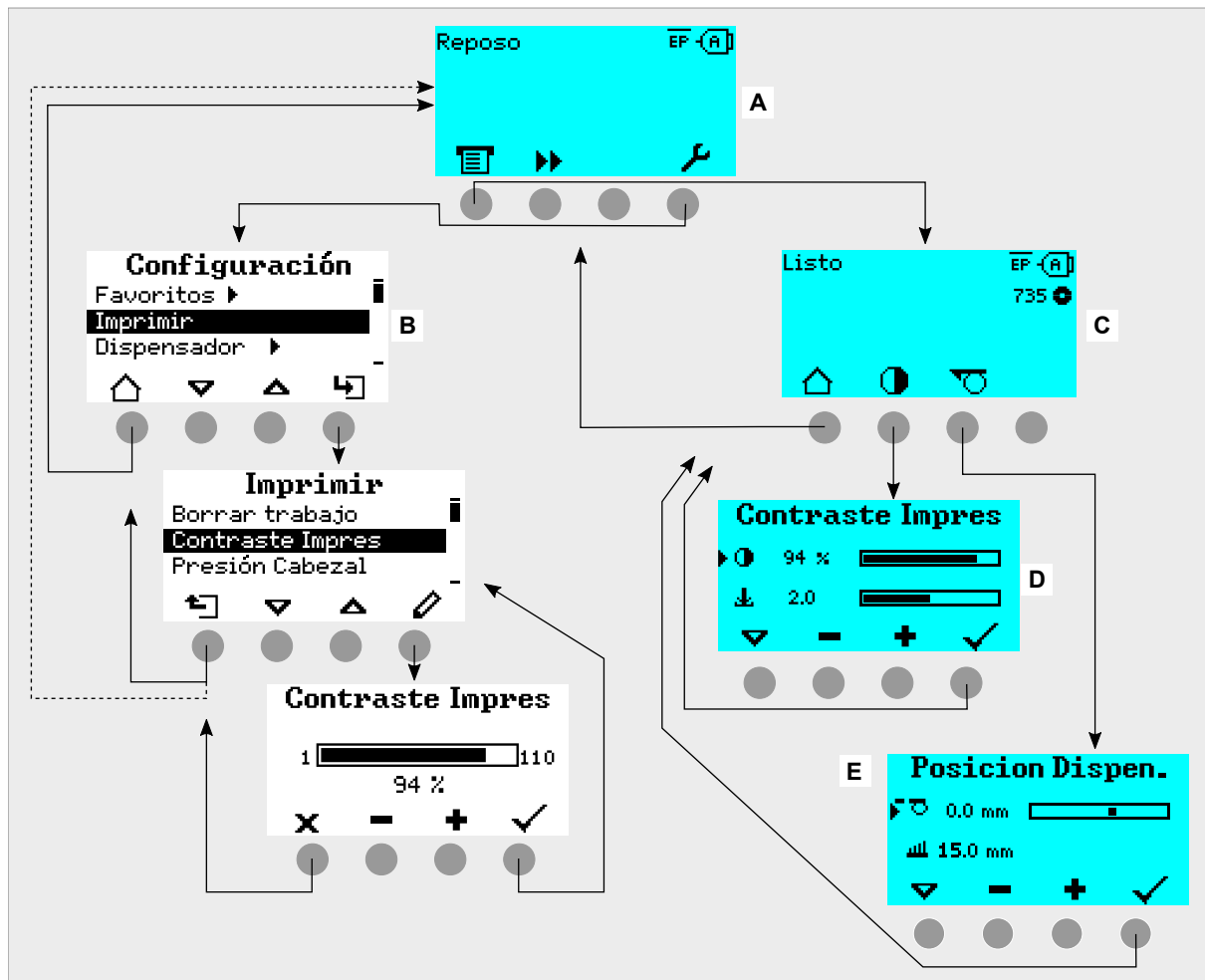
Figura 20: Cambio entre las pantallas: A «Reposo» (cyan), B «Configuración» (blanco), C «Listo» (cyan).
