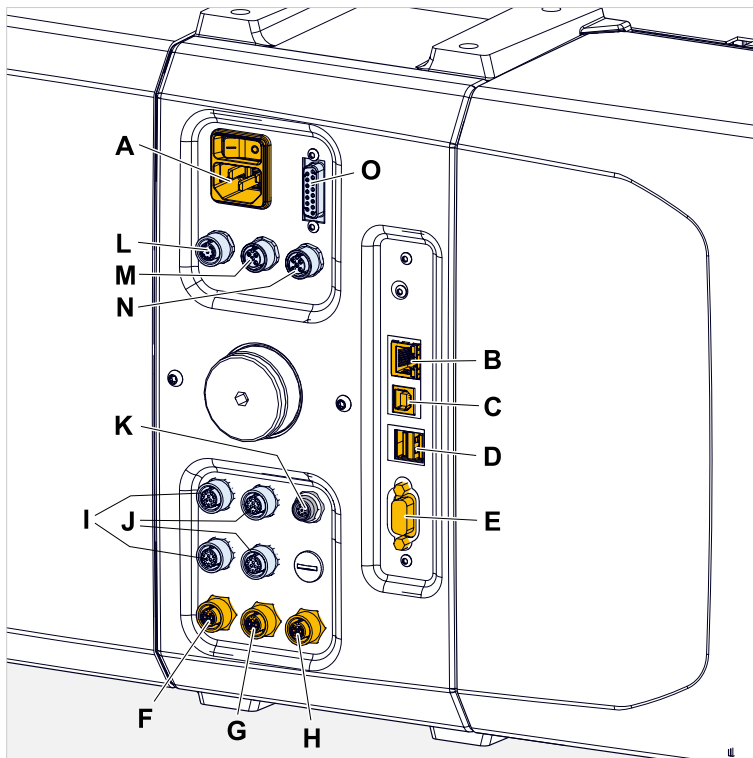
Figura 35: Conexiones en un XPA 94x (naranja = estándar; azul = opcional).
