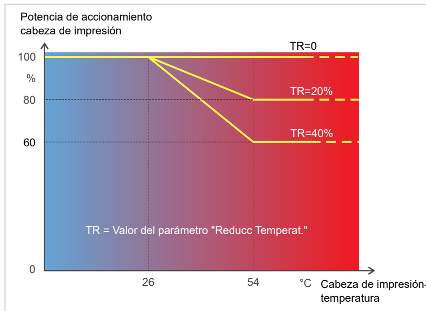
Figura 51: Con el parámetro Sistema > Cntrol Impresion > Reducc Temperat. activado se reduce la potencia del cabezal de impresión - y con ello, indirectamente, el contraste de impresión. La reducción comienza a partir de una temperatura de 26°C. A partir de 54°C se mantiene el valor máximo.
