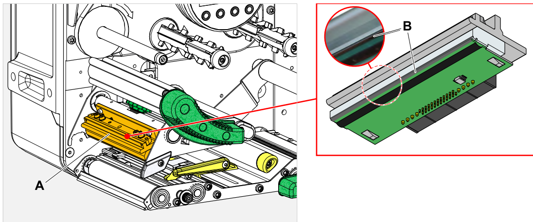
Figura 67: A: Cabezal de impresión, B: Termobarra en el cabezal de impresión
