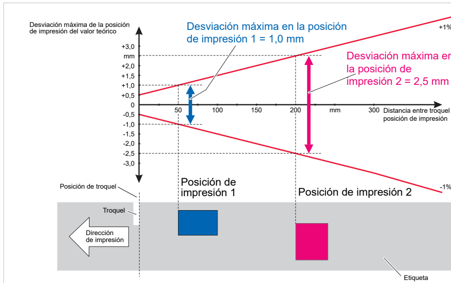
Figura 14: Dependencia de la precisión de huella de la posición de impresión en la etiqueta.
