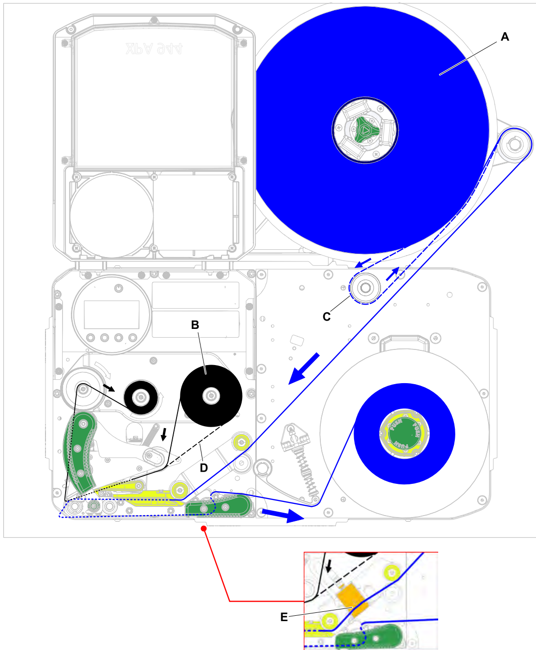
Figura 40: Esquema de enhebrado para el material de etiquetas (A) y lámina de termotransferencia (B) en el XPA 944 LH con desenrollador montado en la parte superior derecha . C = Camino del material de etiquetas enrollado hacia el interior alrededor del rodillo de inversión opcional (aquí necesario); D = Camino de la lámina enrollada con el lado del color hacia el exterior; E = Flujo de material a través del sensor de etiquetas opcional para etiquetas transparentes.
