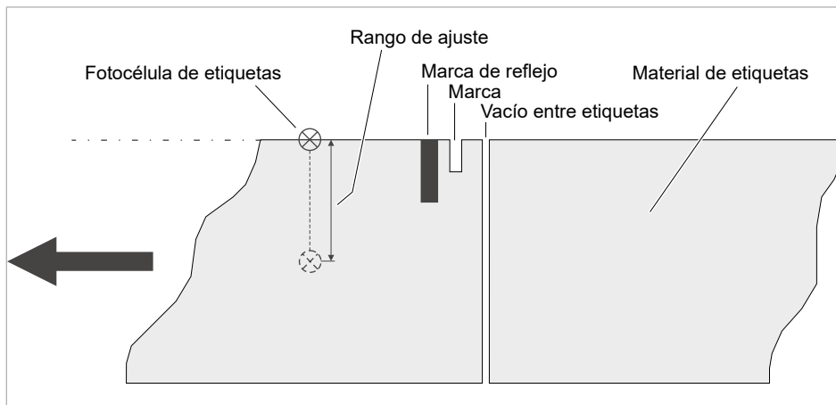
Figura 15: Rango de ajuste de la fotocélula de etiquetas.
