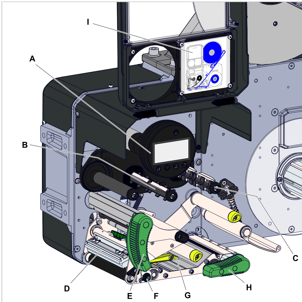
Figura 18: Piezas de mando en el módulo de impresión del XPA 944 LH.
