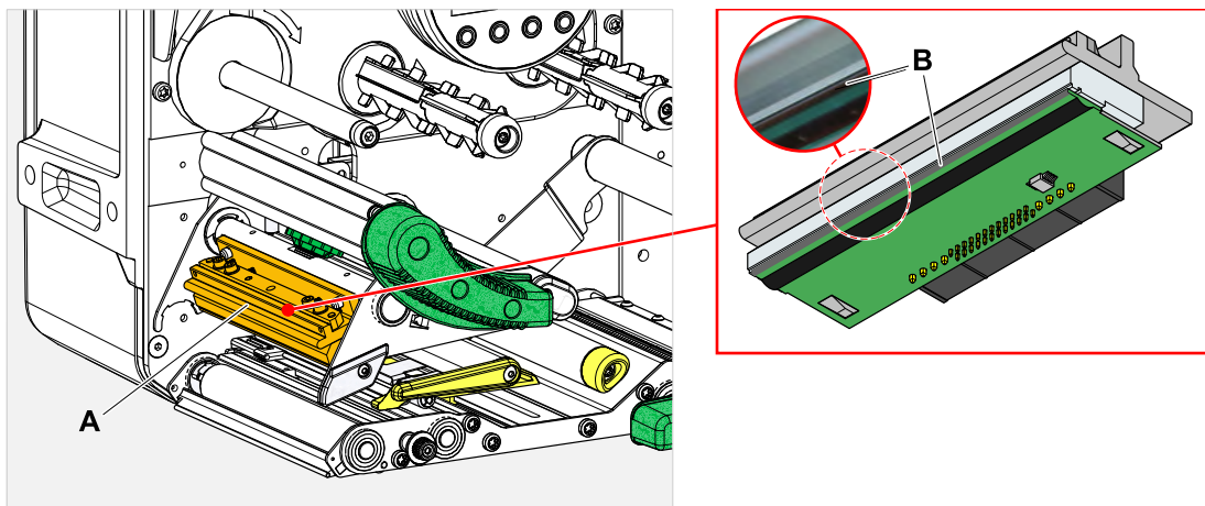
Figura 72: A: Cabezal de impresión, B: Termobarra en el cabezal de impresión
