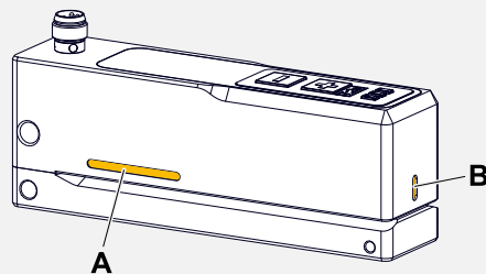
Figura 46: Marcas (A, B) del área de detección en la horquilla del sensor.
