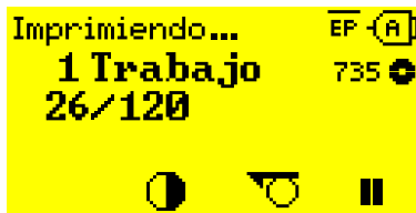
Figura 64: Aviso de fin de lámina durante un trabajo de impresión: El fondo es amarillo, el símbolo de lámina parpadea.
