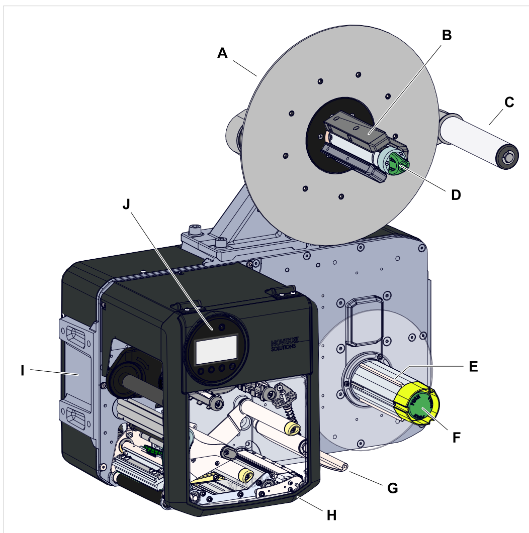
Kép 17: A balkezes XPA 944 kezelőelemei.
