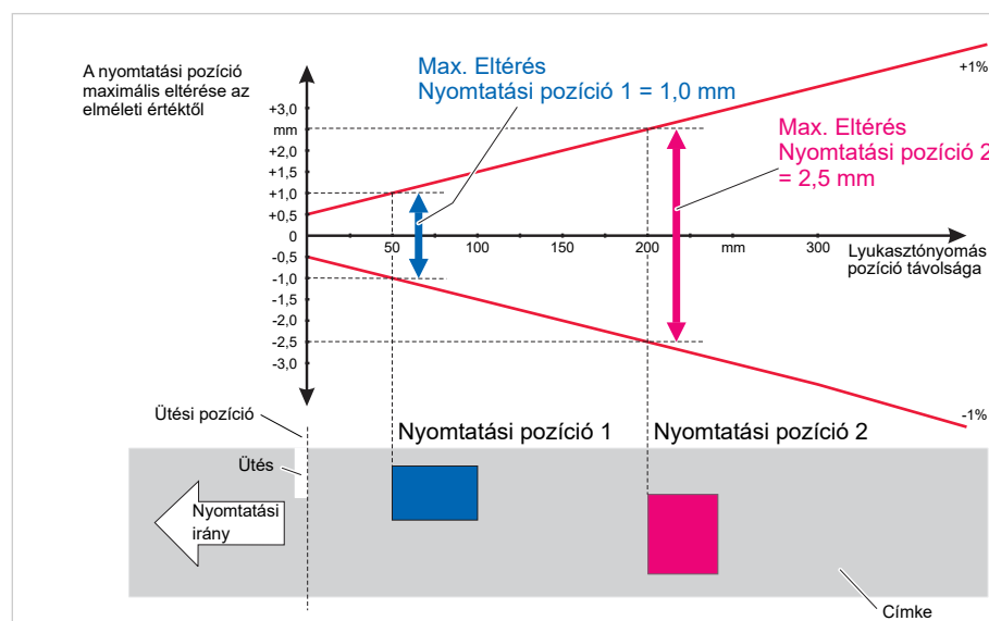
Kép 14: A benyomási pontosság a nyomtatási helyzet függvényében a címkén.
