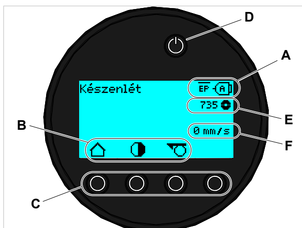
Kép 19: A XPA 94x kezelőmezőjének elemei: A ikonok, amelyek a portok kiosztásáról informálnak, B ikonok, amelyek a billentyűk kiosztását jelzik, C Kezelőgombok, D Standby-gomb, E Fóliatartalék kijelzése, F Szállítószalag sebességének kijelzése (aktivált APSF funkcióval).
