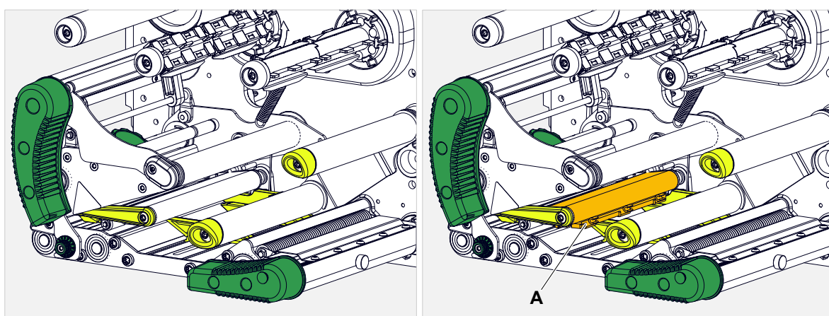
Bild 9: Bal oldalon: XPA 94x Standard; Jobb oldalon: XPA 94x RFID (A: antenna).
