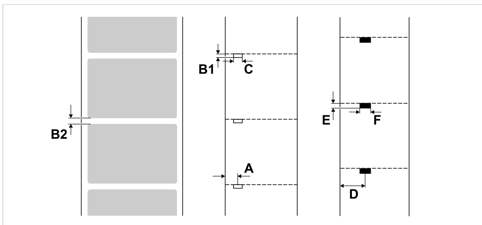
Kép 13: A lyukasztások és fényvisszaverő jelek méretei és helyzete (A: Ütési pozíció, B: Lyukasztási hossz, C: Lyukasztási szélesség, D: Reflexjel pozíciója, E: Fényvisszaverő jel hossza, F: Fényvisszaverő jel szélessége).
