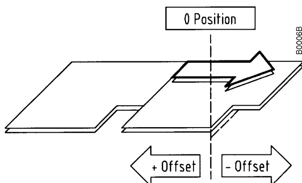
Kép 34: Pozitív és negatív eltolás az előtolás irányához viszonyítva (nyíl).
