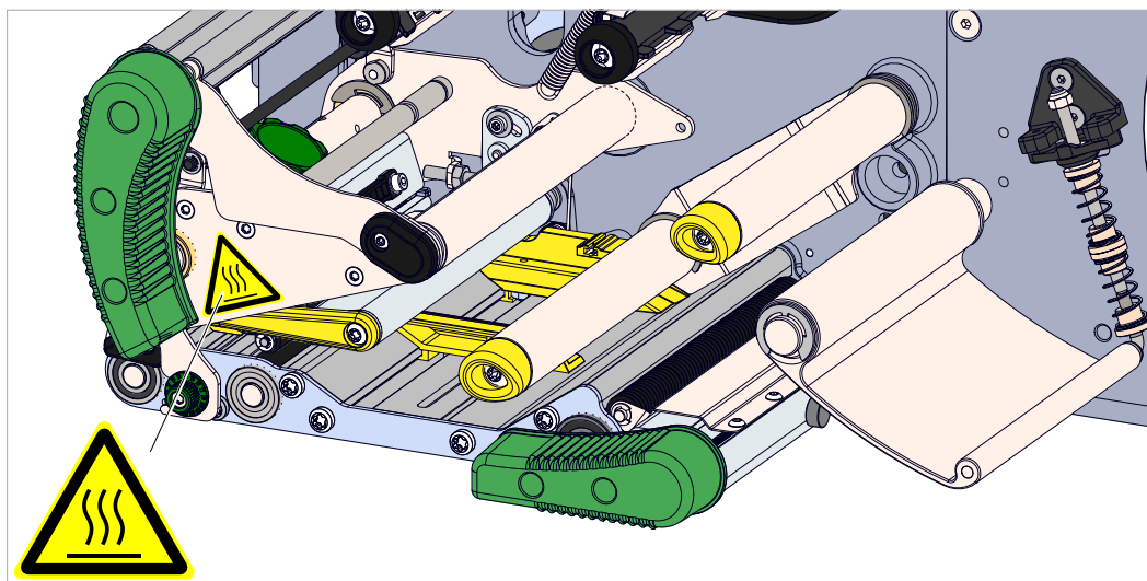
Kép 3: Figyelmeztetési utasítás a XPA 94x-n.
