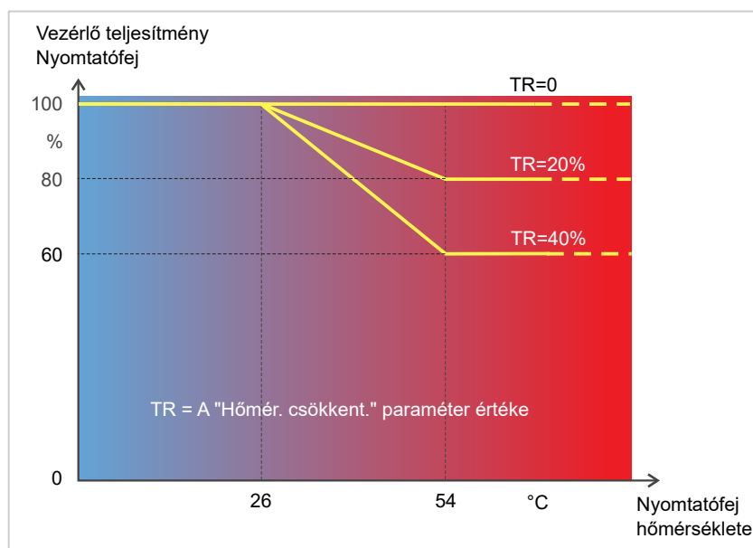
Kép 53: A Rendszer > Nyomatásvezérl. > Hőmér. csökkent. paraméter aktiválásával csökkent a nyomtatófej vezérlési teljesítménye - és ezáltal indirekt módon a nyomtatás kontrasztja. A csökkentés 26°C hőmérséklettől kezdődik. 54°C-tól megőrzi a maximális értéket.
