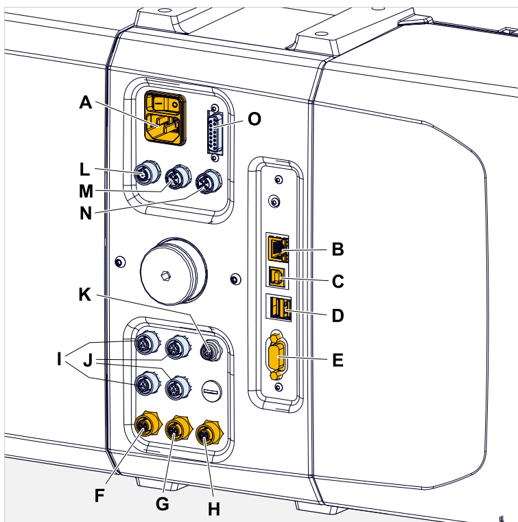
Kép 36: Csatlakoztatás egy XPA 93x-hoz (narancssárga = standard; kék = opció).
