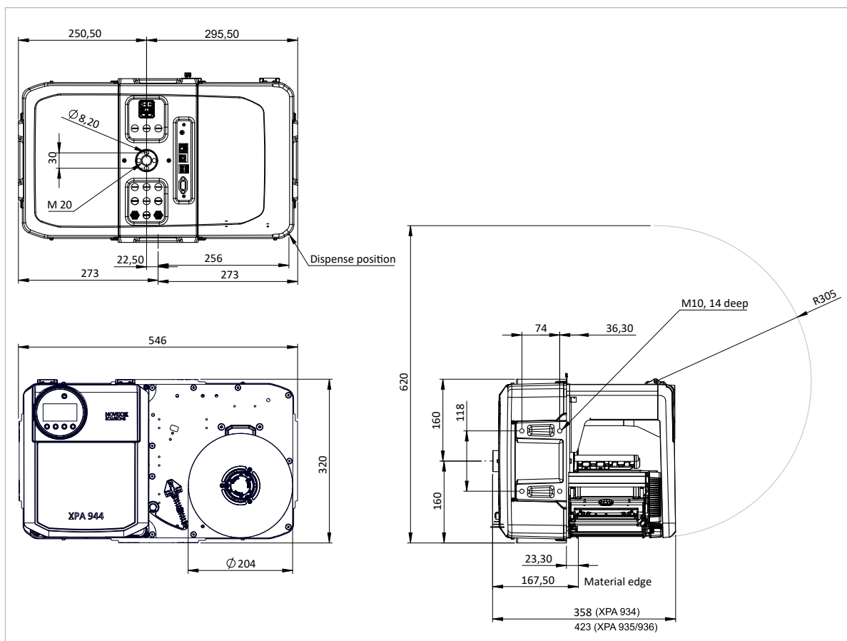
Kép 10: A balkezes XPA 944 méretei.
