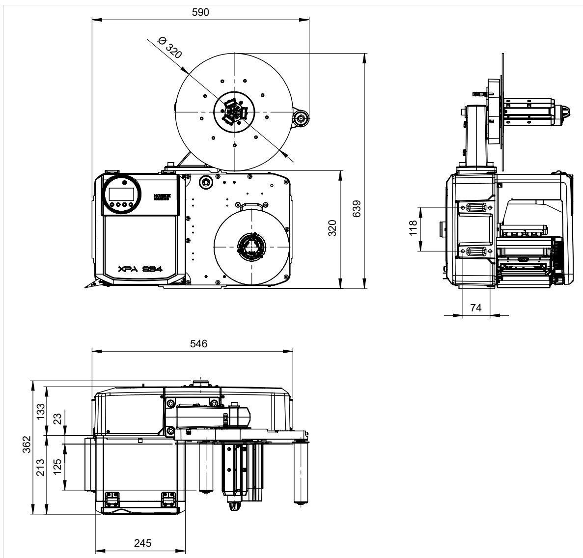
Kép 11: Az XPA 944 LH méretei, anyagletekítővel a jobb felső sarokban.
