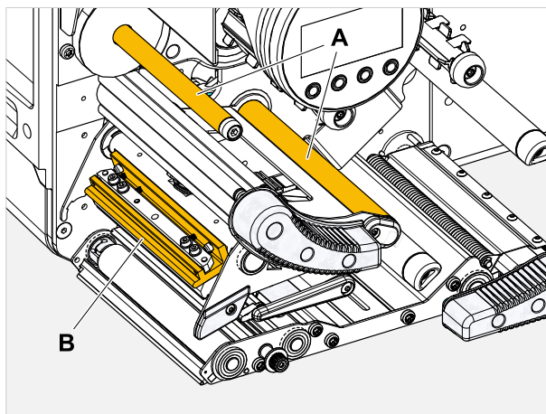
Kép 68: Fóliaeltérítése a XPA 93x esetében (A: eltérítő tengelyek, B: csőr a nyomtatófejnél).
