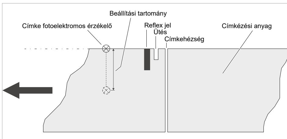
Kép 15: A címkeérzékelő beállítási tartománya.
