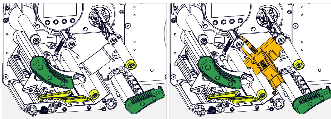
Kép 7: Balra: XPA 94x standard; Jobbra: XPA 94x címkeérzékelővel átlátszó címkékhez.
