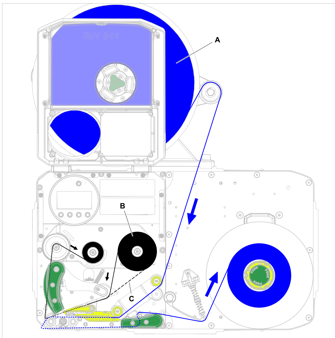
Kép 43: A címkeanyag (A) és a hőtranszferfólia (B) befűzési sémája a balkezes XPA 944-nél lecsévéelővel és balra mutató karral. Ezzel a konfigurációval nem lehet befele csévélte címkeanyagot használni. C = Útvonal a színes oldallal kívül felcsévélte fólia számára.
