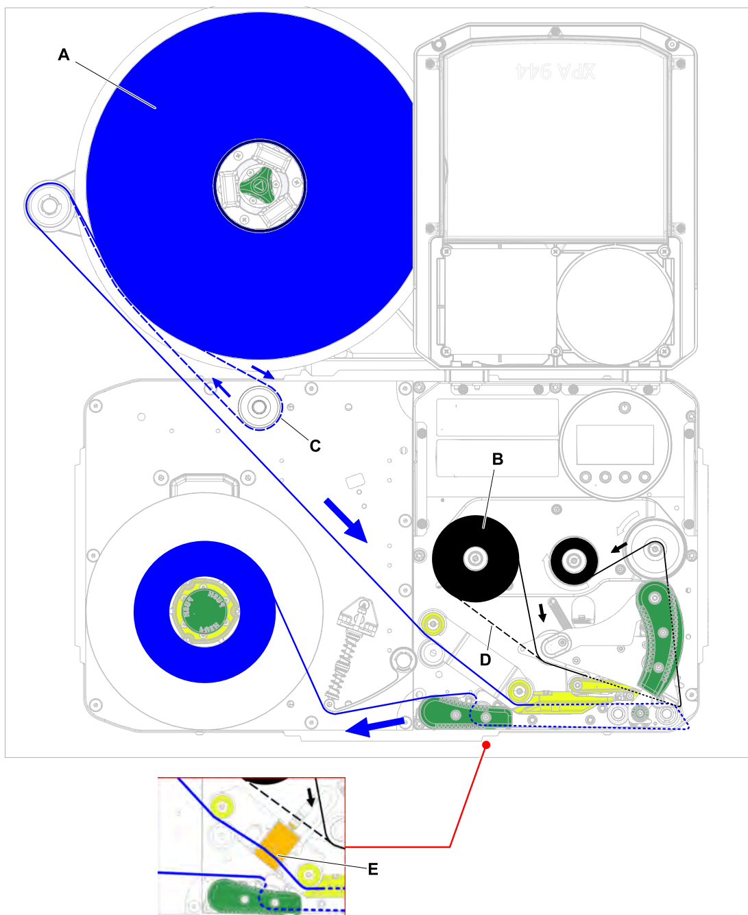
Kép 45: A címkeanyag (A) és a hőtranszferfólia (B) befűzési sémája a jobbkezes XPA 944-nél lecsévéllővel és balra mutató karral. C = Útvonal a befelé csévélt címkeanyag számára az (itt szükséges) opciós terelőgörgő körül, D = útvonal a színes oldallal kívül felcsévélt fólia számára; E = Anyagfutás opcionális címkeérzékelővel átlátszó címkékhez.
