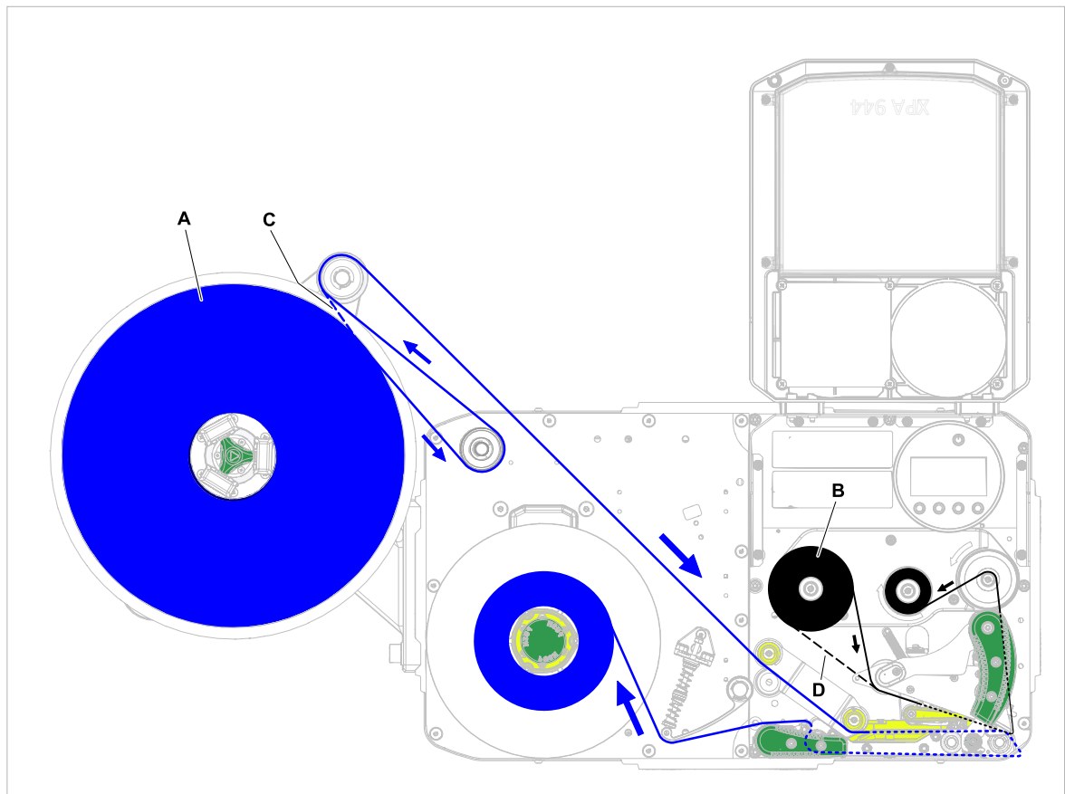
Kép 47: A címkeanyag (A) és a hőtranszferfólia (B) befűzési sémája a jobbkezes XPA 944-nél balra kívül felszerelt lecsévélővel. Ezzel a konfigurációval a kifelé csévélő címkeanyag számára egy opciós terelőgörgő szükséges. C = Útvonal a befelé csévélő címkeanyag számára, D = útvonal a színes oldallal kívül felcsévélő fólia számára.
