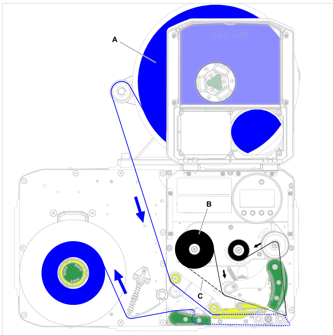
Kép 46: A címkeanyag (A) és a hőtranszferfólia (B) befűzési sémája a jobbkezes XPA 944-nél lecsévélővel és jobbra mutató karral. Ezzel a konfigurációval nem lehet befele csévélte címkeanyagot használni. C = Útvonal a színes oldallal kívül felcsévélte fólia számára.
