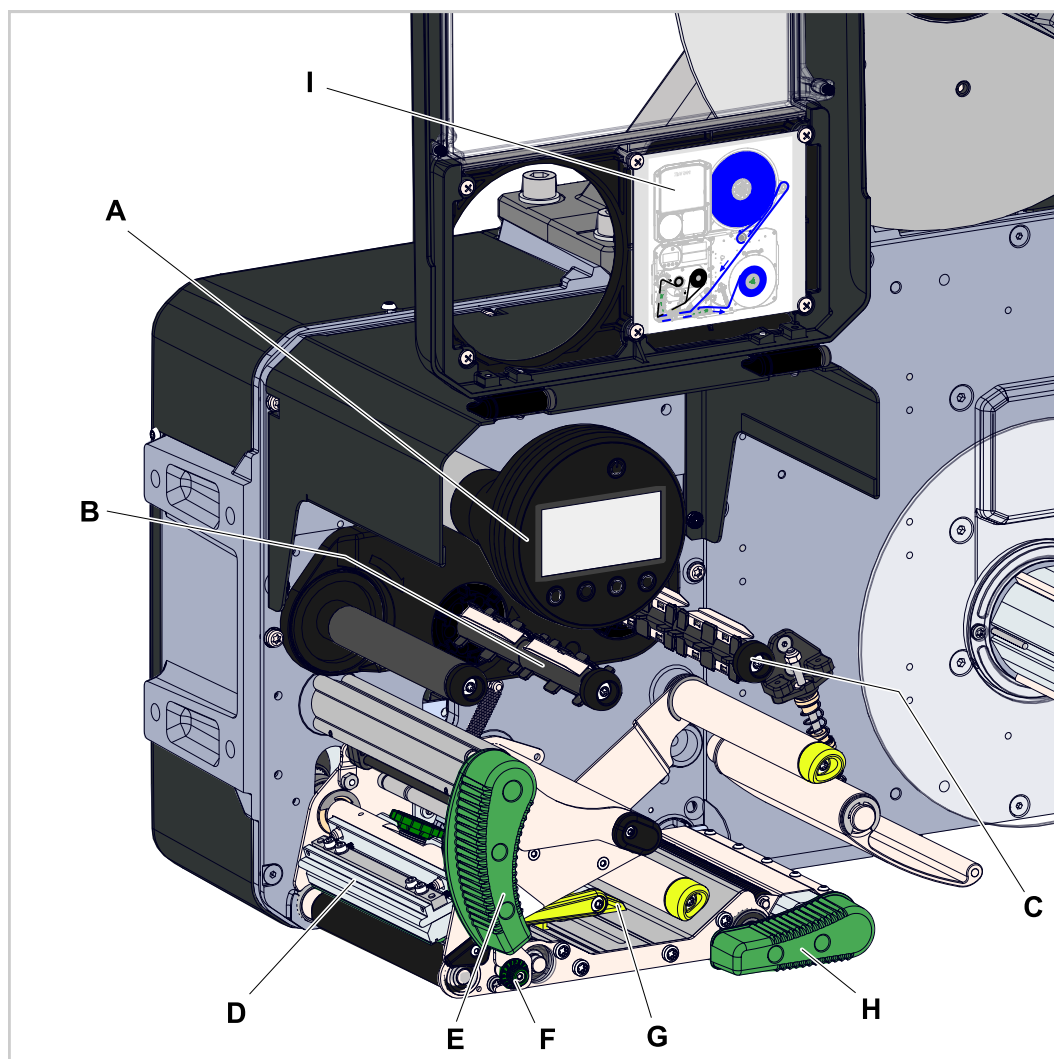
Kép 18: A balkezes XPA 944 kezelőelemei nyomtatómodulnál.
