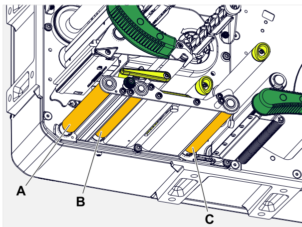
Afbeelding 71: A drukwals, B toevoerwals, C trekwals
