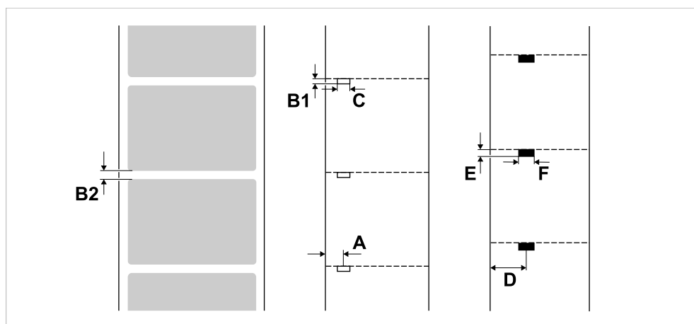
Afbeelding 13: Afmetingen en posities van stansen en reflectiemarkeringen (A: Stanspositie, B: Stanslengte, C: Standsbreedte, D: Reflectiemarkeringspositie, E: Reflectiemarkeringslengte, F: reflectiemarkeringsbreedte).
