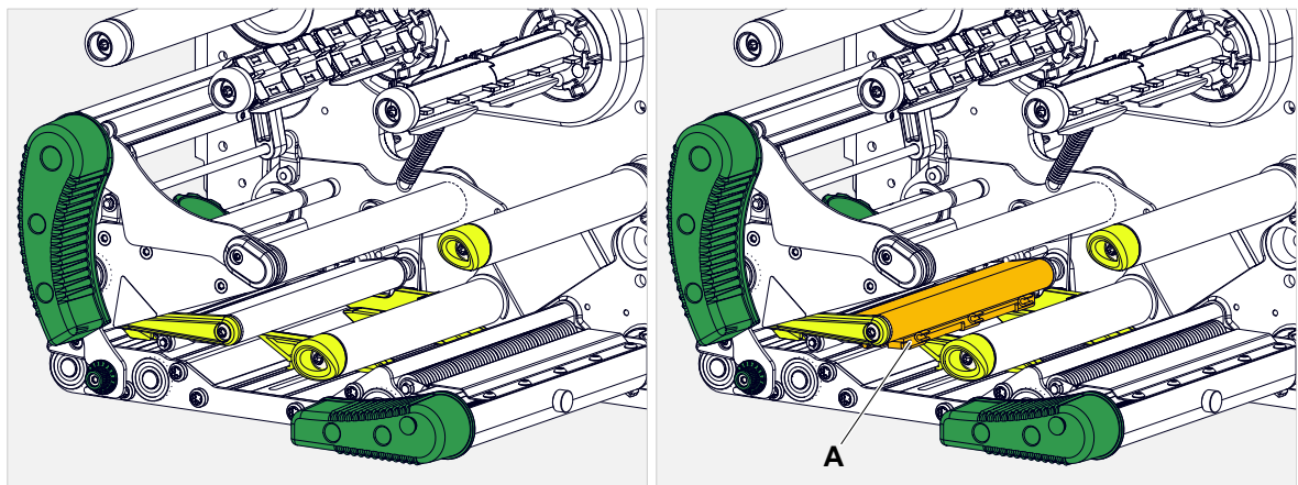
Bild 9: Links: XPA 94x standaard; Rechts: XPA 94x RFID (A: antenne).
