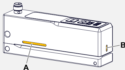
Afbeelding 47: Markeringen (A, B) van het detectiegebied op de sensorgaffel.
