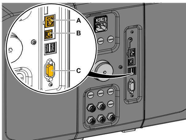
Afbeelding 35: Data-interfaces op XPA 94x (A ethernet, B USB, C RS 232).
