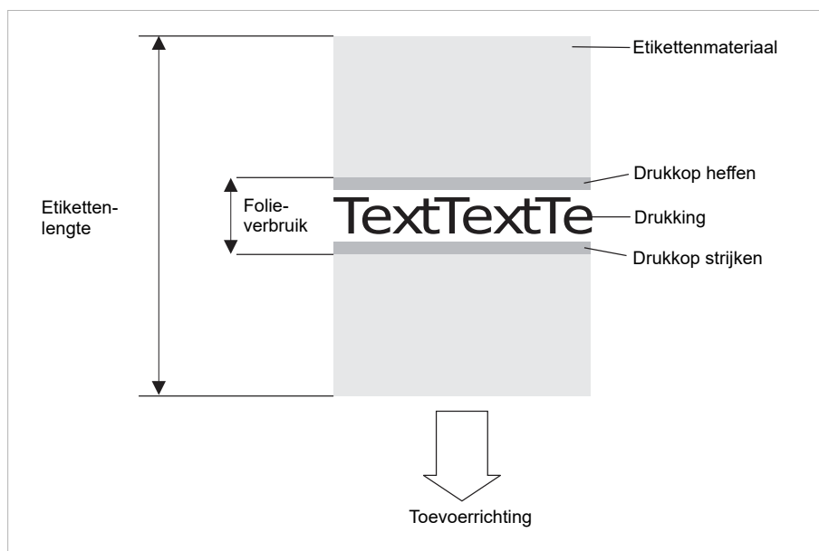
Afbeelding 6: Folieverbruik voor etiketten met kleine drukzone bij ingeschakelde foliespaar-automatiek. Het folieverbruik is in geringe mate hoger dan de lengte van het bedrukte bereik.
