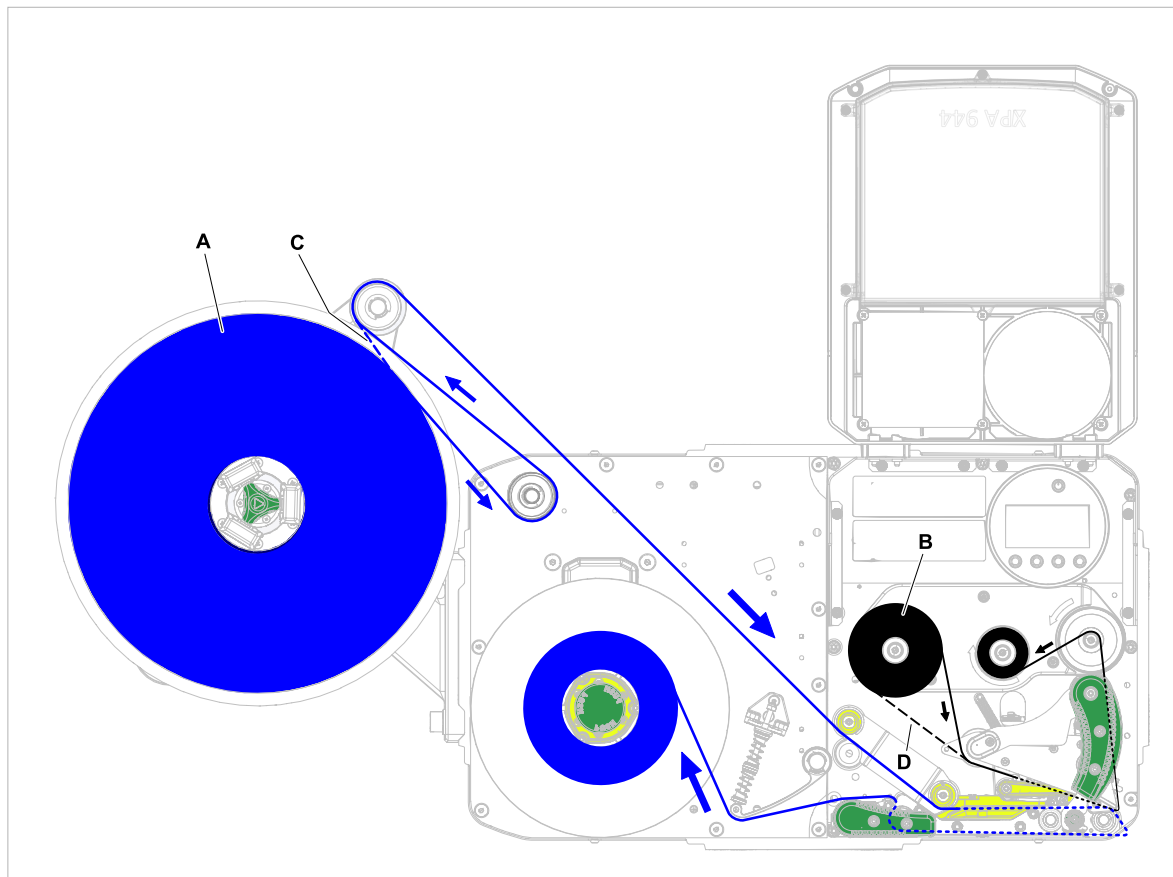
Afbeelding 45: Rijgschema voor etikettenmateriaal (A) en thermo transfer-folie (B) op XPA 944 RH met afwikkelaar "Pro 300" links buiten gemonteerd. Met deze configuratie is voor naar buiten gewikkeld etikettenmateriaal een optionele omkeerrol vereist. C = pad voor naar binnen gewikkeld etikettenmateriaal; D = pad voor met de kleurzijde naar buiten gewikkelde folie.
