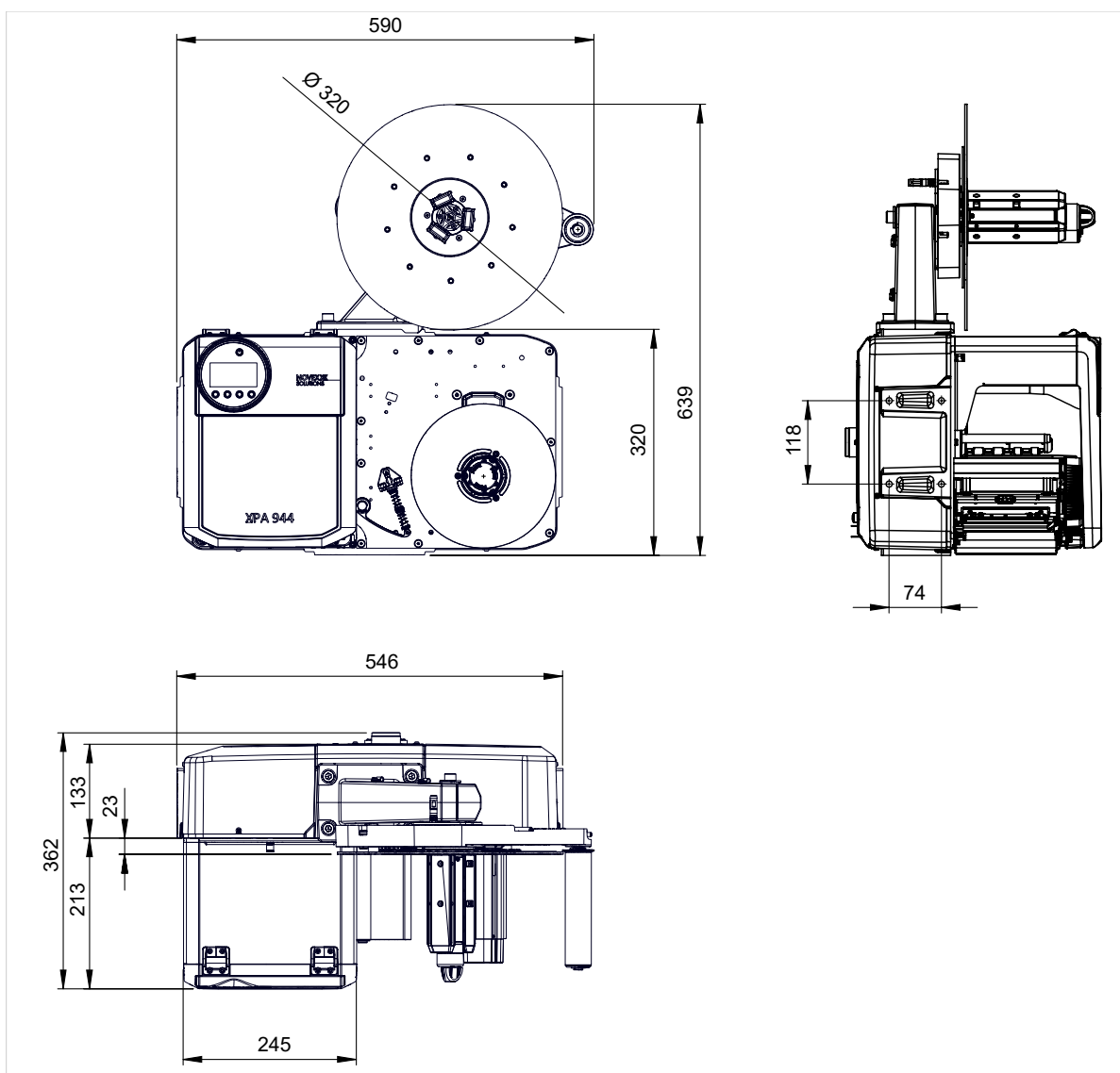
Afbeelding 11: Afmetingen van de XPA 944 LH met materiaalaftrekker rechtsboven.
