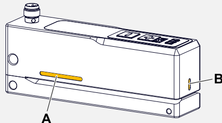
Afbeelding 46: Markeringen (A, B) van het detectiegebied op de sensorgaffel.
