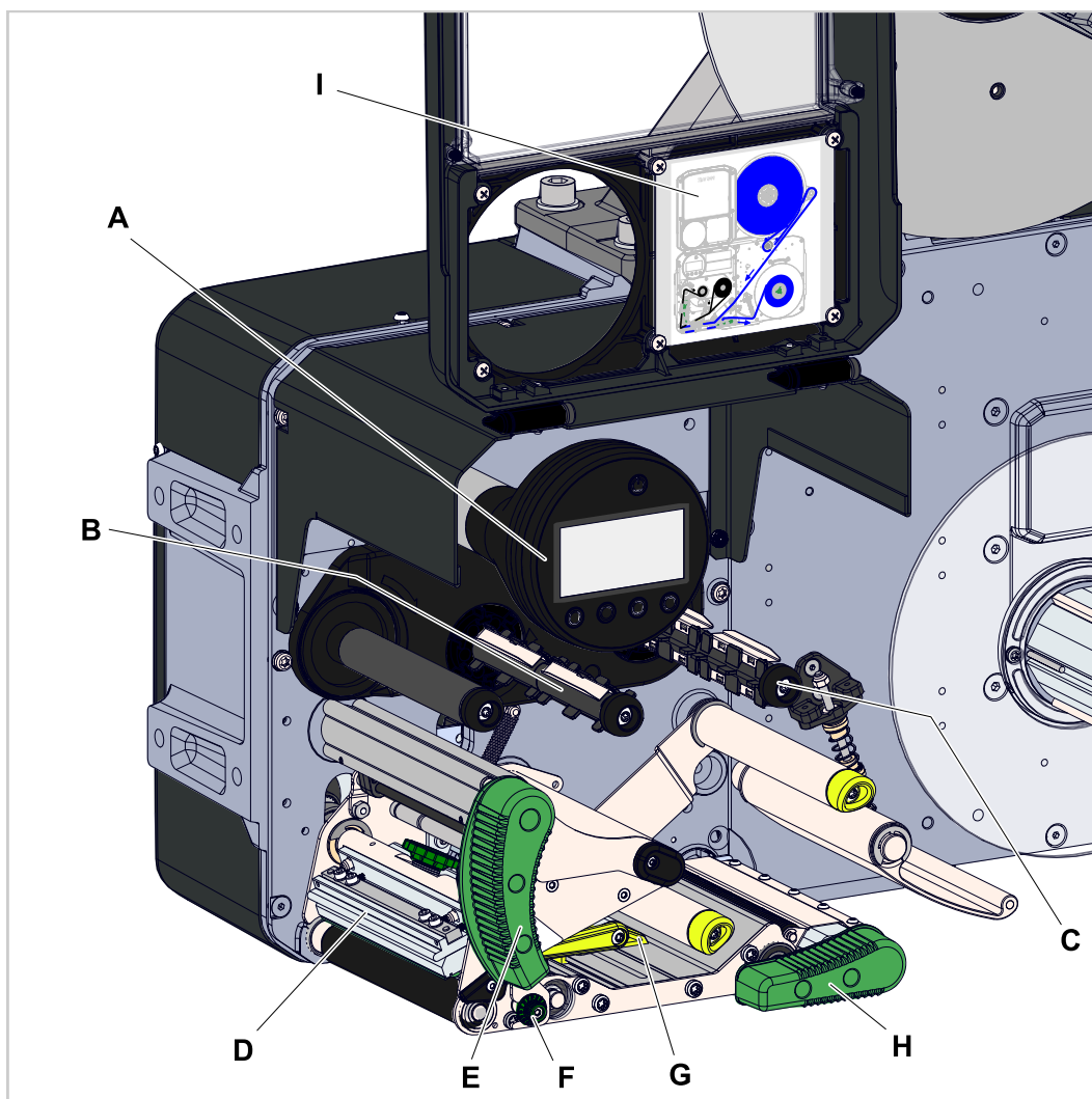
Afbeelding 17: Bedieningsdelen op printmodule van XPA 944 LH.
