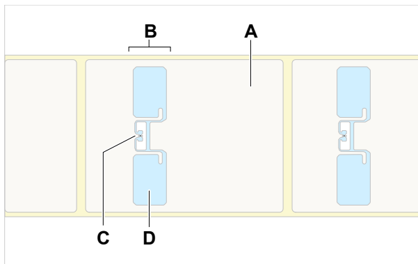
Bild 8: Schematische weergave van een RFID-label (A: label, B: transponder, C: chip, D: antenne)
