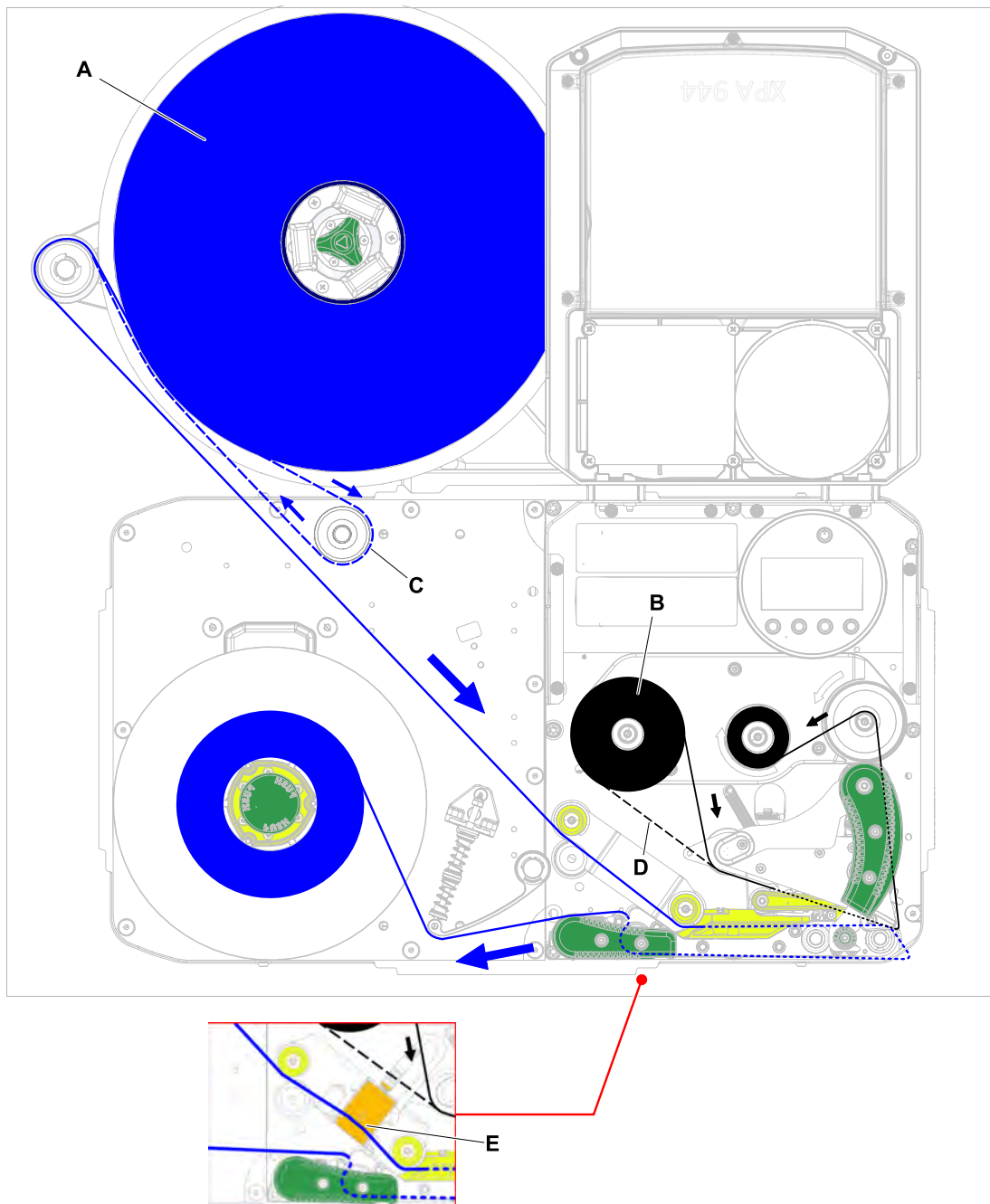
Afbeelding 43: Rijgschema voor etikettenmateriaal (A) en thermo transfer-folie (B) op XPA 944 RH met afwikkelaar met naar links gerichte arm. C = pad voor naar binnen gewikkeld etikettenmateriaal om de (hier vereiste) optionele omkeerrol; D = pad voor met de kleurzijde naar buiten gewikkelde folie; E = Materiaalstroom door de optionele labelsensor voor transparante etiketten.
