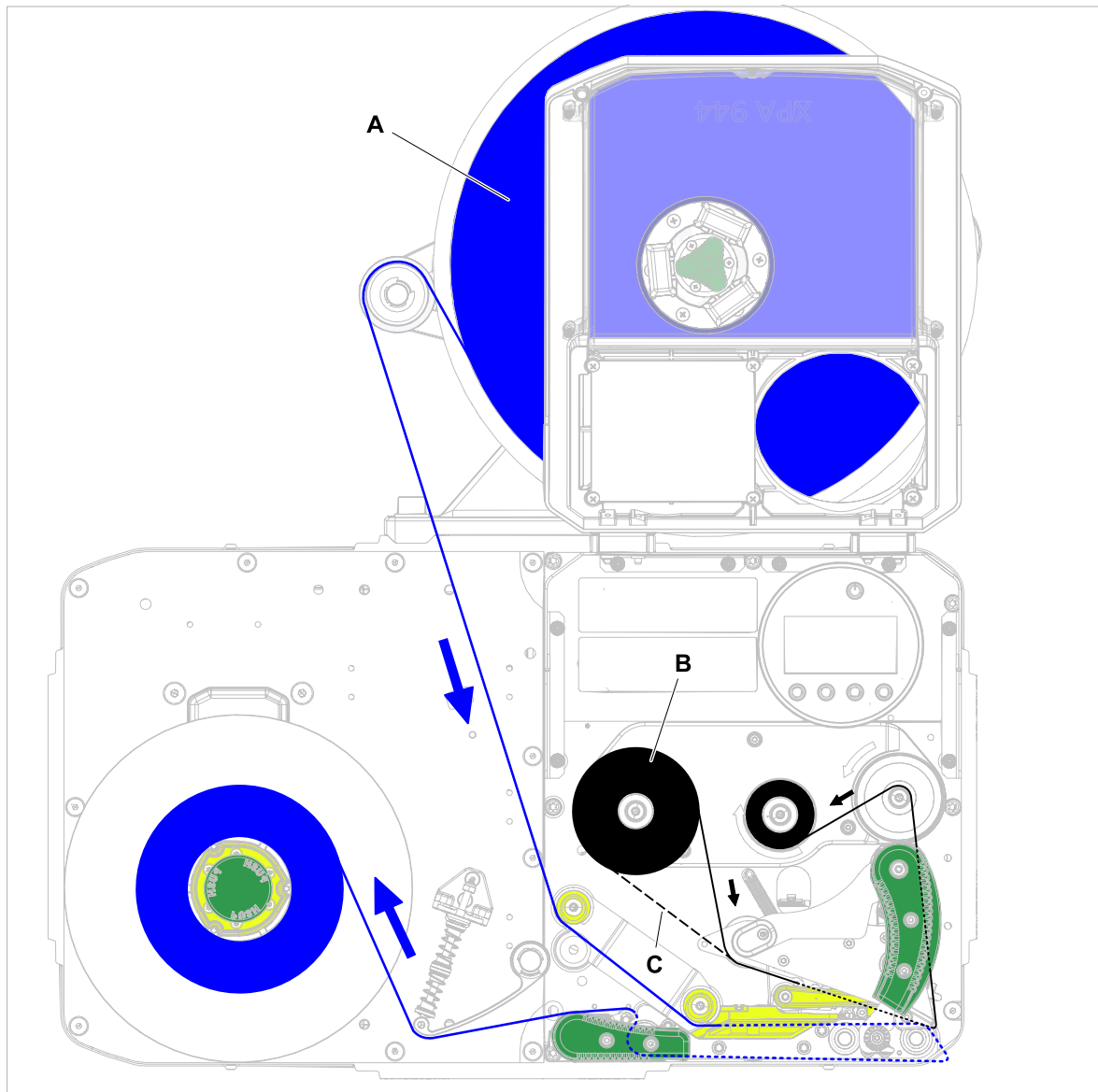
Afbeelding 44: Rijdschema voor etikettenmateriaal (A) en thermo transfer-folie (B) op XPA 944 RH met afwikkelaar "Pro 300" met naar rechts gerichte arm. Naar binnen gewikkeld etikettenmateriaal kan met deze configuratie niet worden gebruik. C = pad voor met de kleurzijde naar buiten gewikkelde folie.
