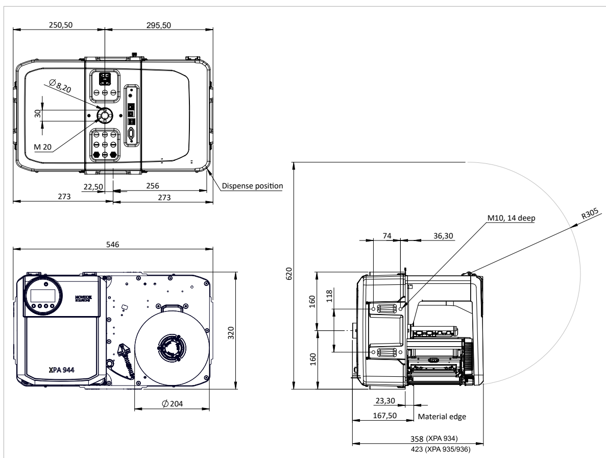
Afbeelding 10: Afmetingen van XPA 944 LH.
