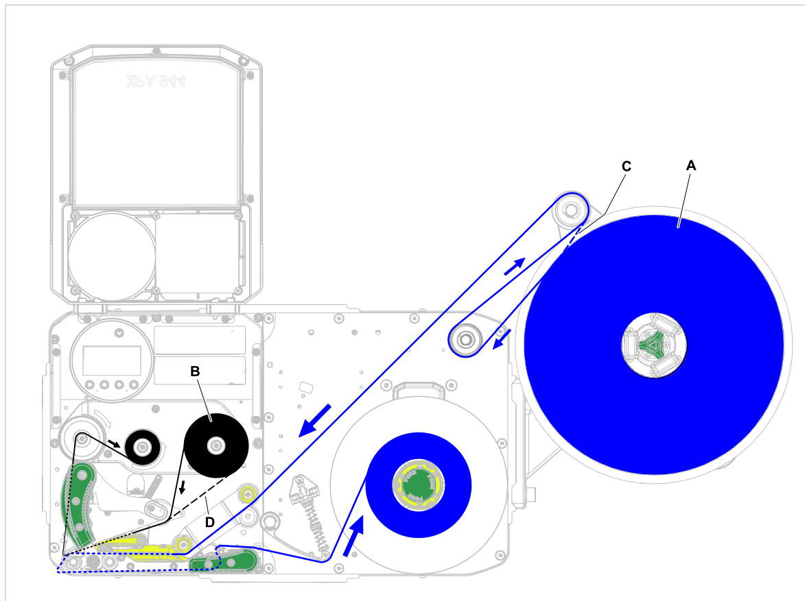
Afbeelding 42: Rijgschema voor etikettenmateriaal (A) en thermo transfer-folie (B) op XPA 944 LH met afwikkelaar "Pro 300" rechts buiten gemonteerd. Met deze configuratie is voor naar buiten gewikkeld etikettenmateriaal een optionele omkeerrol vereist. C = pad voor naar binnen gewikkeld etikettenmateriaal; D = pad voor met de kleurzijde naar buiten gewikkelde folie.
