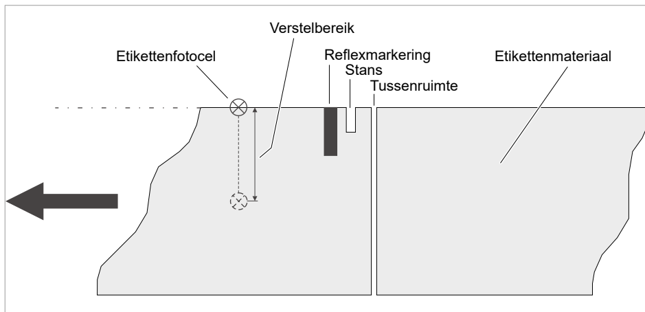
Afbeelding 15: Verstellbereik van etikettenfotocel.
